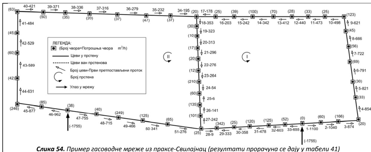
Слика 54. Пример гасоводне мреже из праксе-Свилајнац (резултати прорачуна се дају у табели 41)
