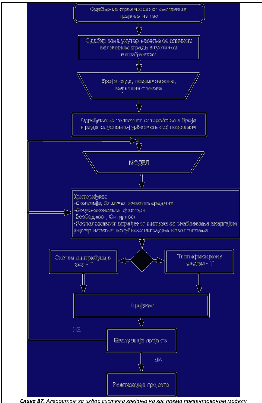
Слика 87. Алгоритам за избор система грејања на гас према презентованом моделу
