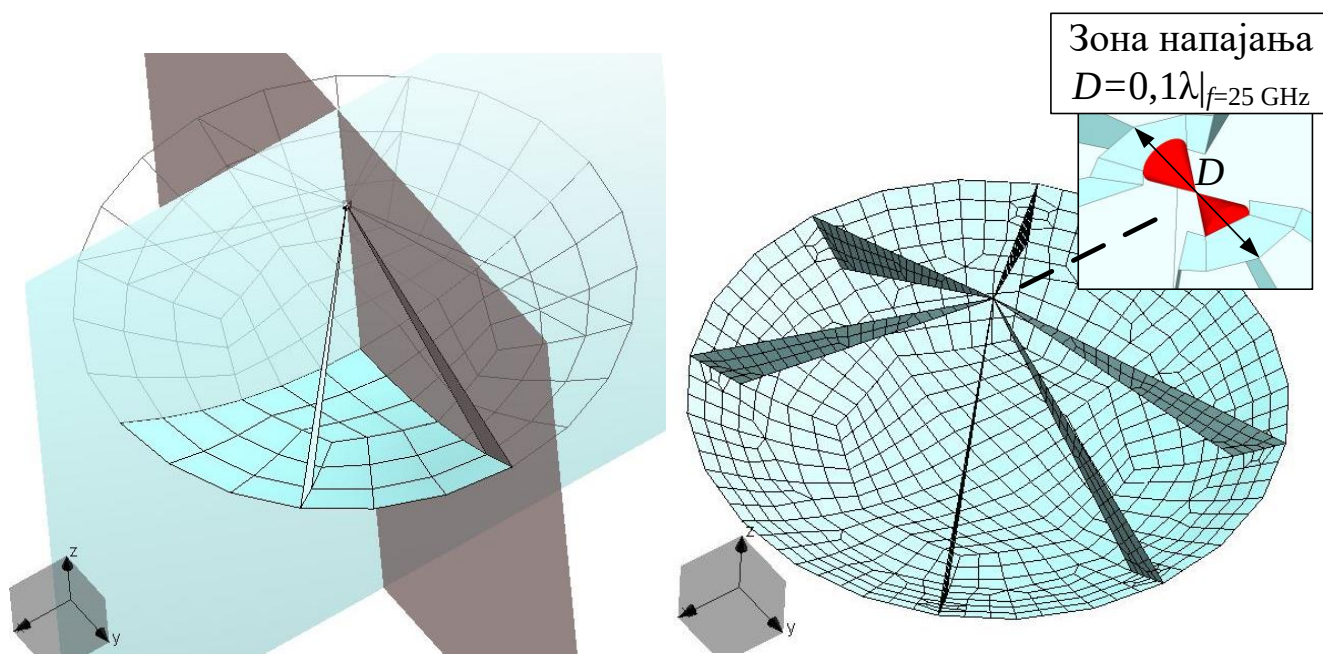
Слика 3.6. Пример нумеричког модела IRA-е са традиционалним краковима; подела на четрвоуглове и увеличани приказ зоне напајања.
