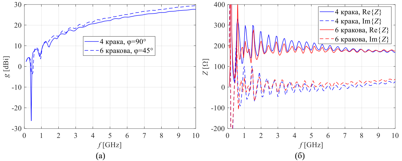
Слика 3.17. Поређење IRA са 4 крака и \phi = 40^\circ са IRA са 6 кракова по а) појачању [35], и б) импеданси [35].
