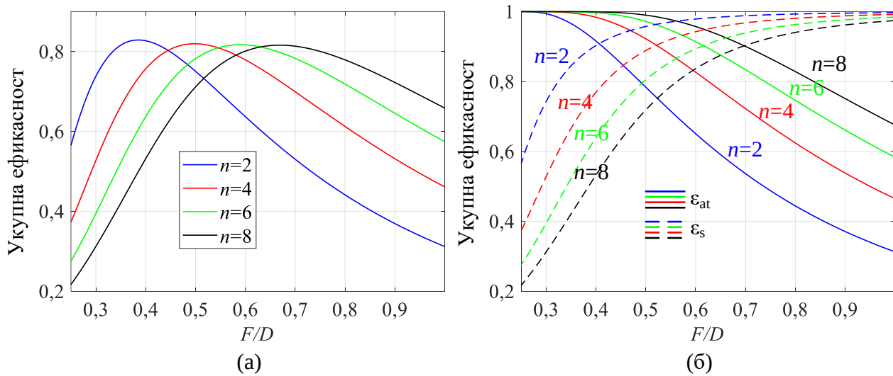
Слика 2.3. а) Израчуната ефикасност као функција F/D за неколико ширина главног снопа примарног радијатора дефинисаног кроз (2.11). б) Графички приказ компромиса између високог \varepsilon_{at} и високог \varepsilon_s који се мора постићи како би се постигла максимална ефикасност.
