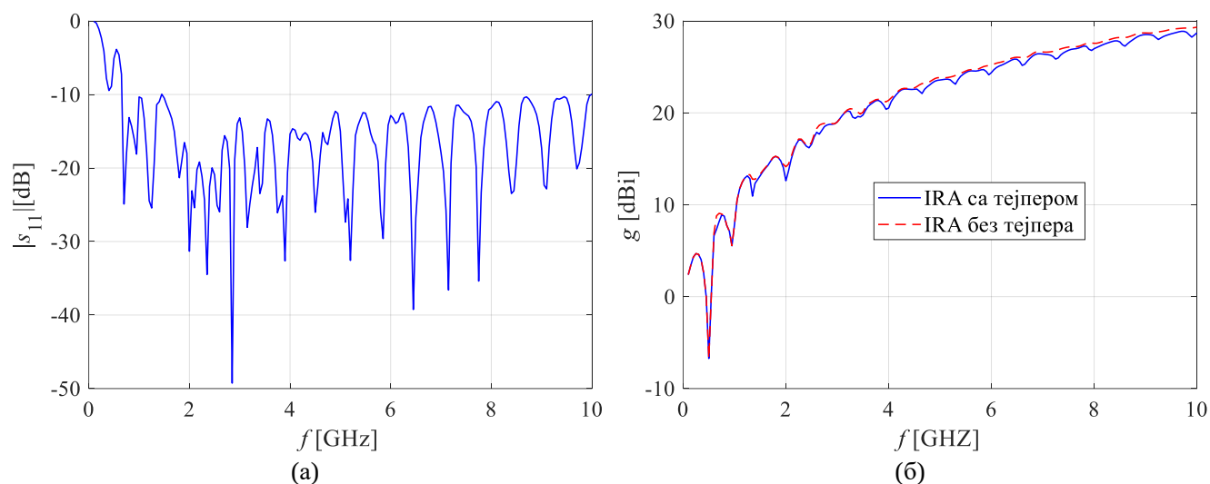
Слика 4.11. Резултати за а) коефицијент рефлексије и б) појачање антене моделоване заједно са тејпером [35].
