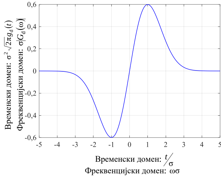
Слика 3.21. Облик диференцираног Гаусовог импулса и његов амплитудски спектар.
