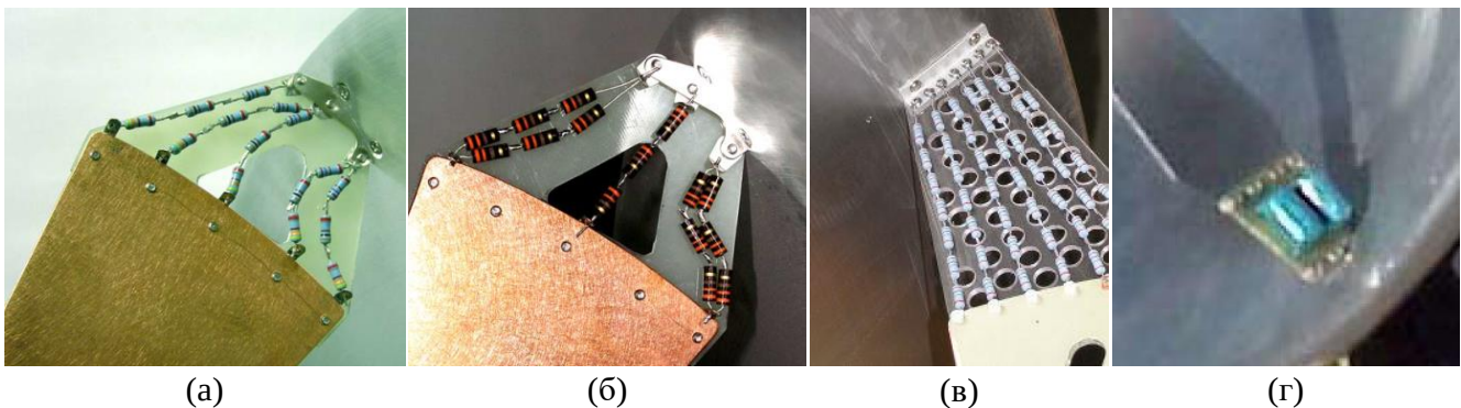
Слика 2.11. Отпорници за терминисање кракова. а) Мрежа од 15 отпорника (3 отпорника повезаних редно, а 5 група у паралелој вези) у технологији танких филмова [49]. б) Мрежа од 15 угљеничних отпорника (3 отпорника повезаних редно, а 5 у паралелој вези) [49]. в) Мрежа са великим бројем отпорника ради повећања максималне снаге IRA-е [50]. г) Висконапонски отпорници (енглески: high voltage resistors, HVR) [48].
