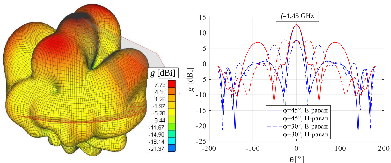
Слика 3.16. Цепање дијаграма зрачења код IRA-е са \phi = 30^\circ на 1,45 GHz.
