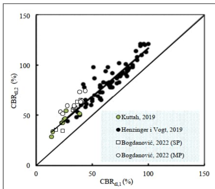
Slika 7.25. Zbirni prikaz između vrednosti CBR_{dl} dobijenih iz privog ( CBR_{dl,1} ) i drugog ( CBR_{dl,2} ) udarca padajućeg teža za krupnozrne materijale i literaturnih podataka
