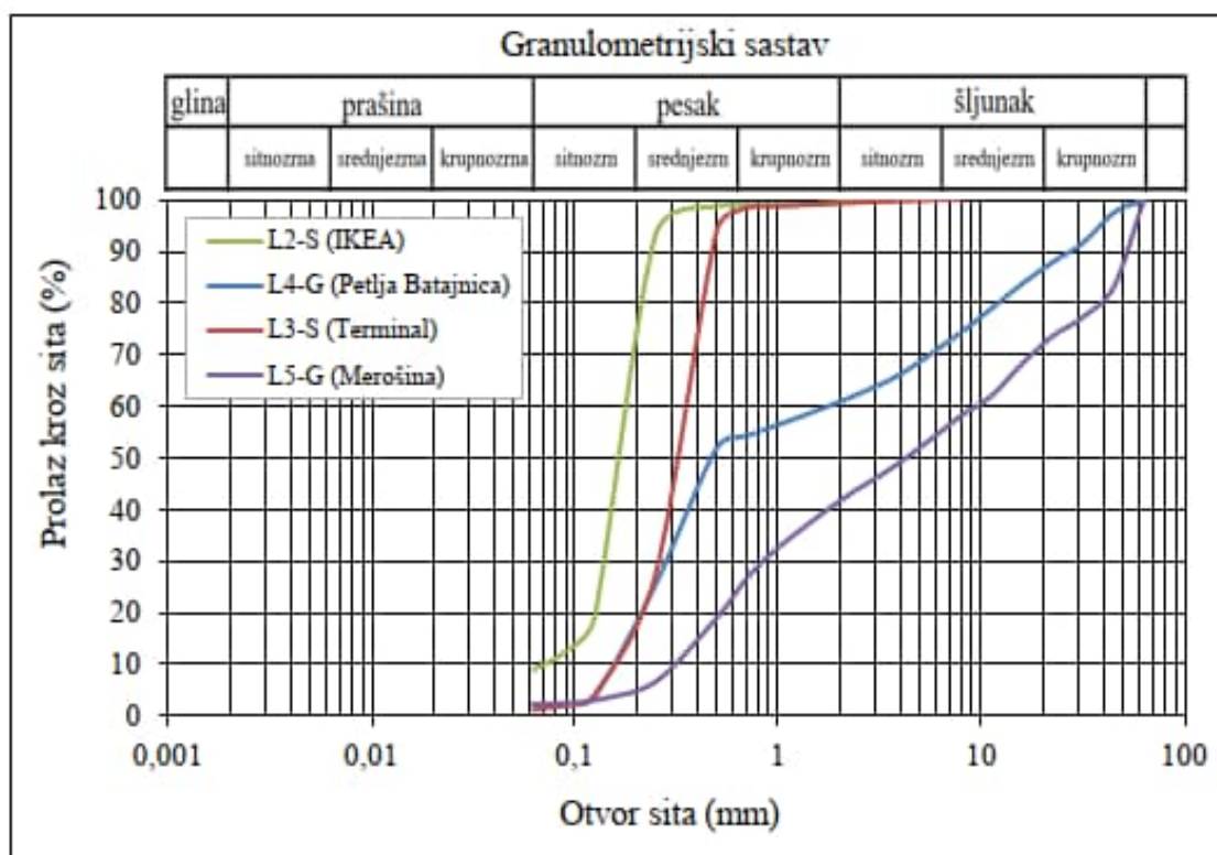
Slika 4.4. Granulometrijski sastav – reprezentativna analiza krupnozrnih materijala
