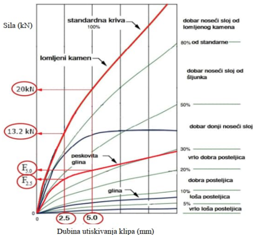
Slika 3.9. Prikaz rezultata CBR vrednosti (S.Maraš-Dragojević, 2022)
