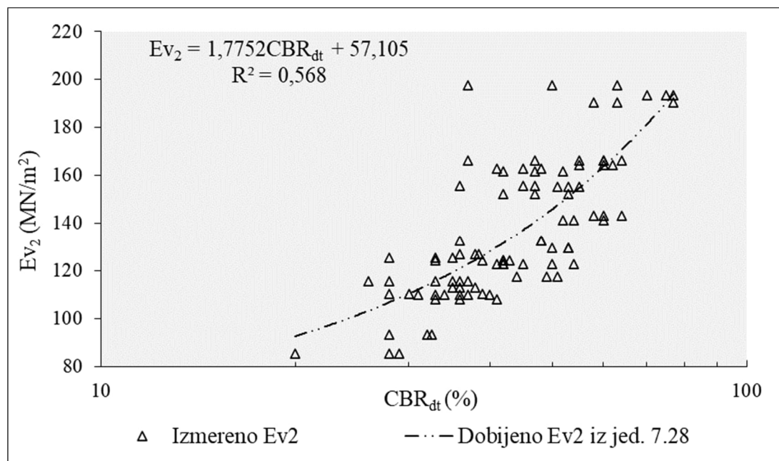
Slika 7.12. Korelaciona zavisnost „in situ“ parametara, modula deformacije E_{v2} i dinamičkog CBR_{dt} na posteljičnom sloju, lokacija L4-G
