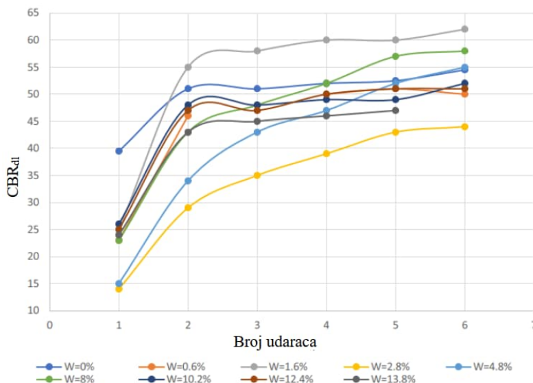
Slika 4.18. Uticaj broja udaraca padajućeg teža na laboratorijske dinamičke vrednosti CBR_{dl} pri različitim sadržajima vode peskovitog uzorka (Dina Kuttah, 2019)
