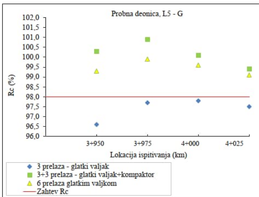
Slika 4.13. Grafički prikaz rezultata stepena zbijenosti ( R_c ) u zavisnosti od broja prelaza valjka (L5-G)
