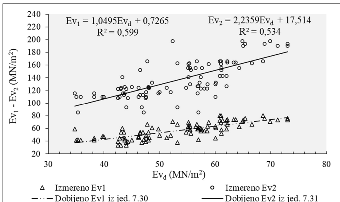
Slika 7.14. Korelaciona zavisnost „in situ“ parametara, modula deformacije E_{v1} - E_{v2} i dinamičkog modula deformacije E_{vd} na posteljičnom sloju, lokacija L4-G
