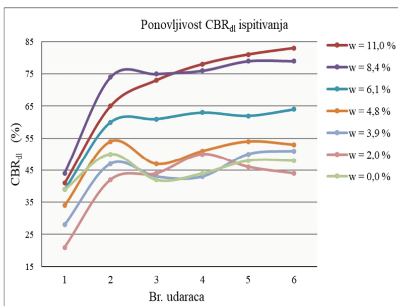
Slika 4.19. Uticaj uzastopnih udaraca padajućeg teža na laboratorijske dinamičke vrednosti CBR_{dl} pri različitim sadržajima vode, L4-G
