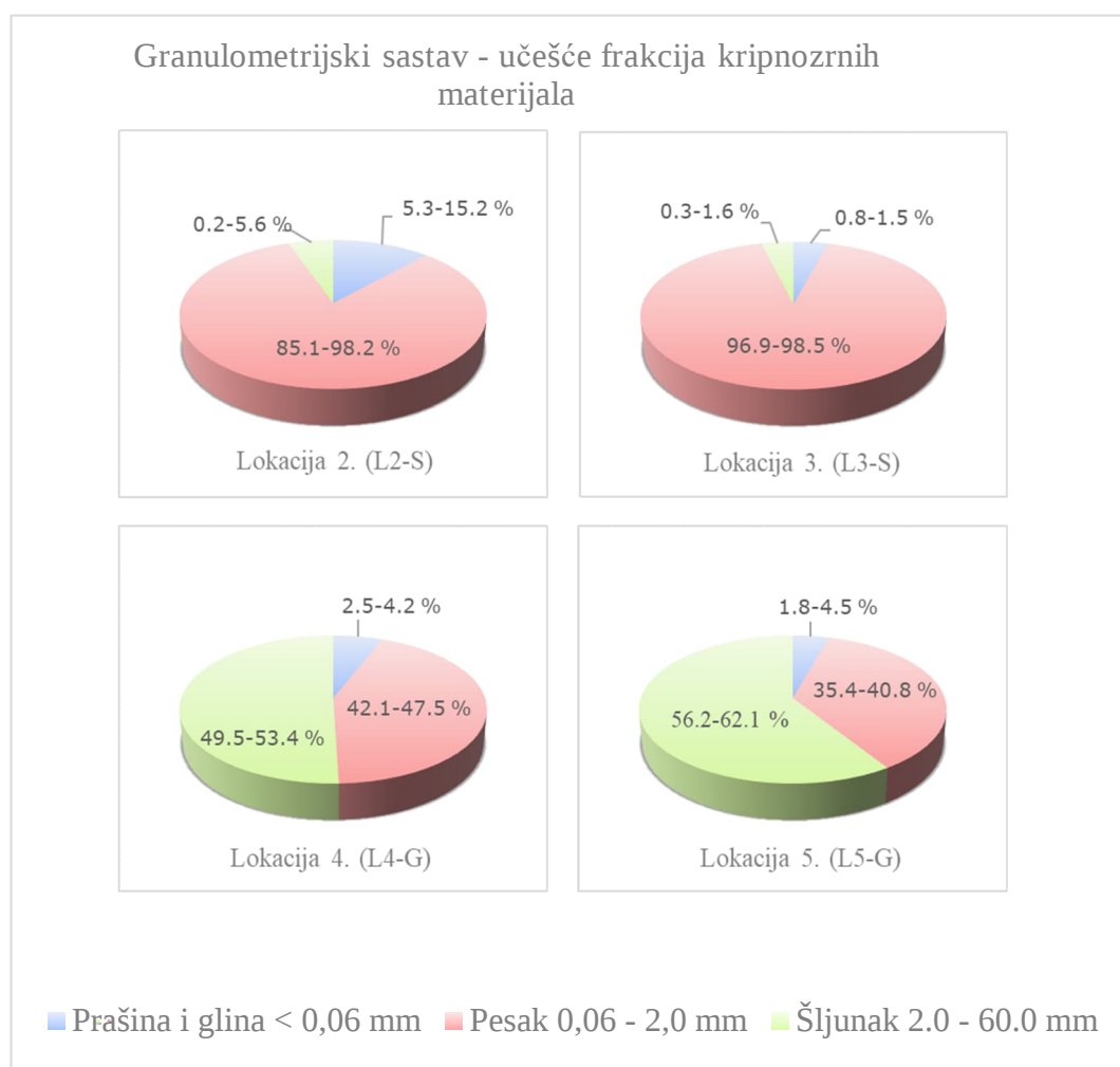
Slika 4.5. Granulometrijski sastav – učešće frakcija krupnozrnih materijala
