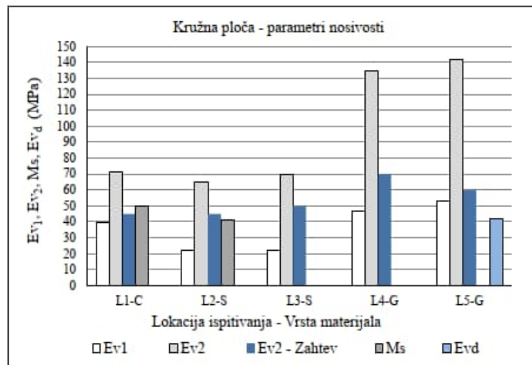
Slika 5.11. Zbirni prikaz srednjih vrednosti parametara nosivosti predmetnih lokacija donjih slojeva saboraćajnica
