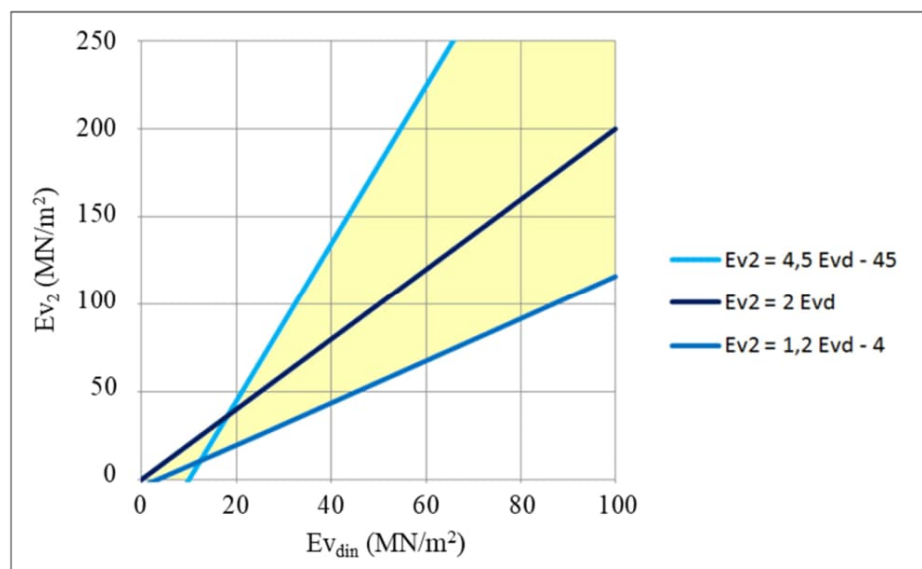
Slika 6.4. Uprošćene korelacione zavisnosti između vrednosti Ev_2 i Ev_{vd} (Lehmann, 2011)
