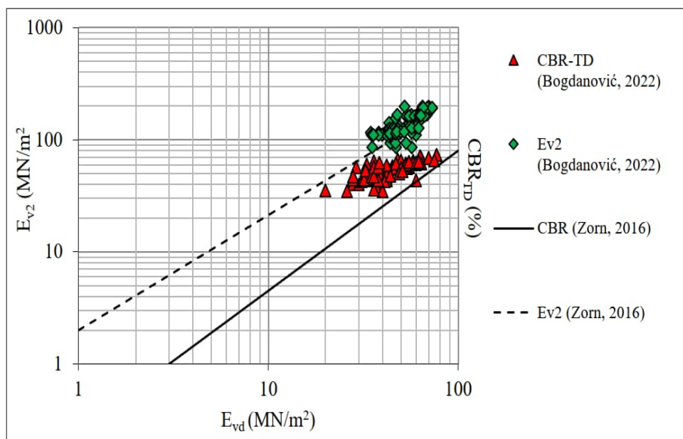
Slika 7.30. Zbirni prikaz parametara dinamičkog modula deformacije E_{vd} , modula deformacije E_{v2} i dinamičkog CBR_{dt} sa literarnim podacima (Zorn, 2016)
