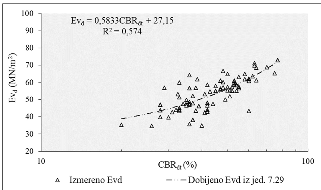
Slika 7.13. Korelaciona zavisnost „in situ“ parametara, dinamičkog modula deformacije E_{vd} i dinamičkog CBR_{dt} na posteljičnom sloju, lokacija L4-G
