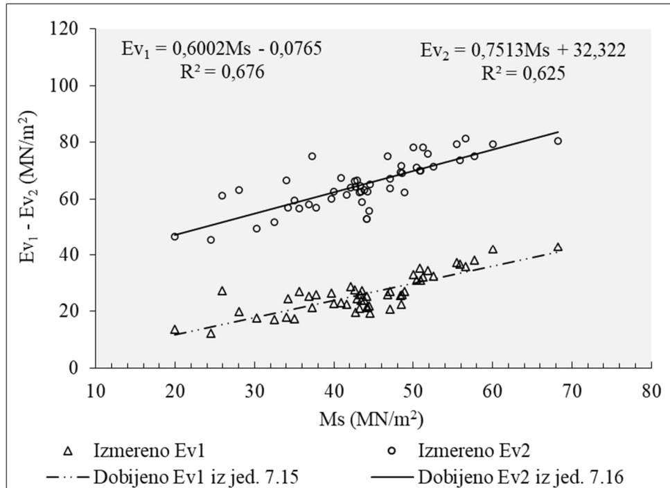
Slika 7.5 Korelaciona zavisnost „in situ“ parametara, modula deformacije E_{v1} - E_{v2} i modula stižljivosti M_s na II sloju nasipa, lokacija L2-S
