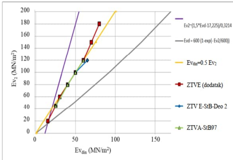
Slika 6.3. Korelacione zavisnosti između vrednosti Ev_2 i Ev_{vd} za sitnozrne i krupnozrne materijale (Lehmann, 2011)
