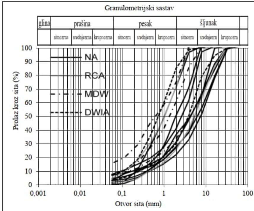
Slika 6.10. Granulometrijski sastav ipitivanih materijala (Henzinger, C. i Vogt, S., 2019)
