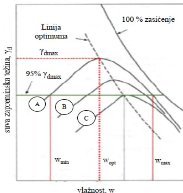
Slika 3.6. Odnos suve zapremine težine ( \gamma_d ) i vlažnosti ( w ) tla, ilustrujući najefikasnije uslove zbijanja „in situ“ (Seed, 1964)
