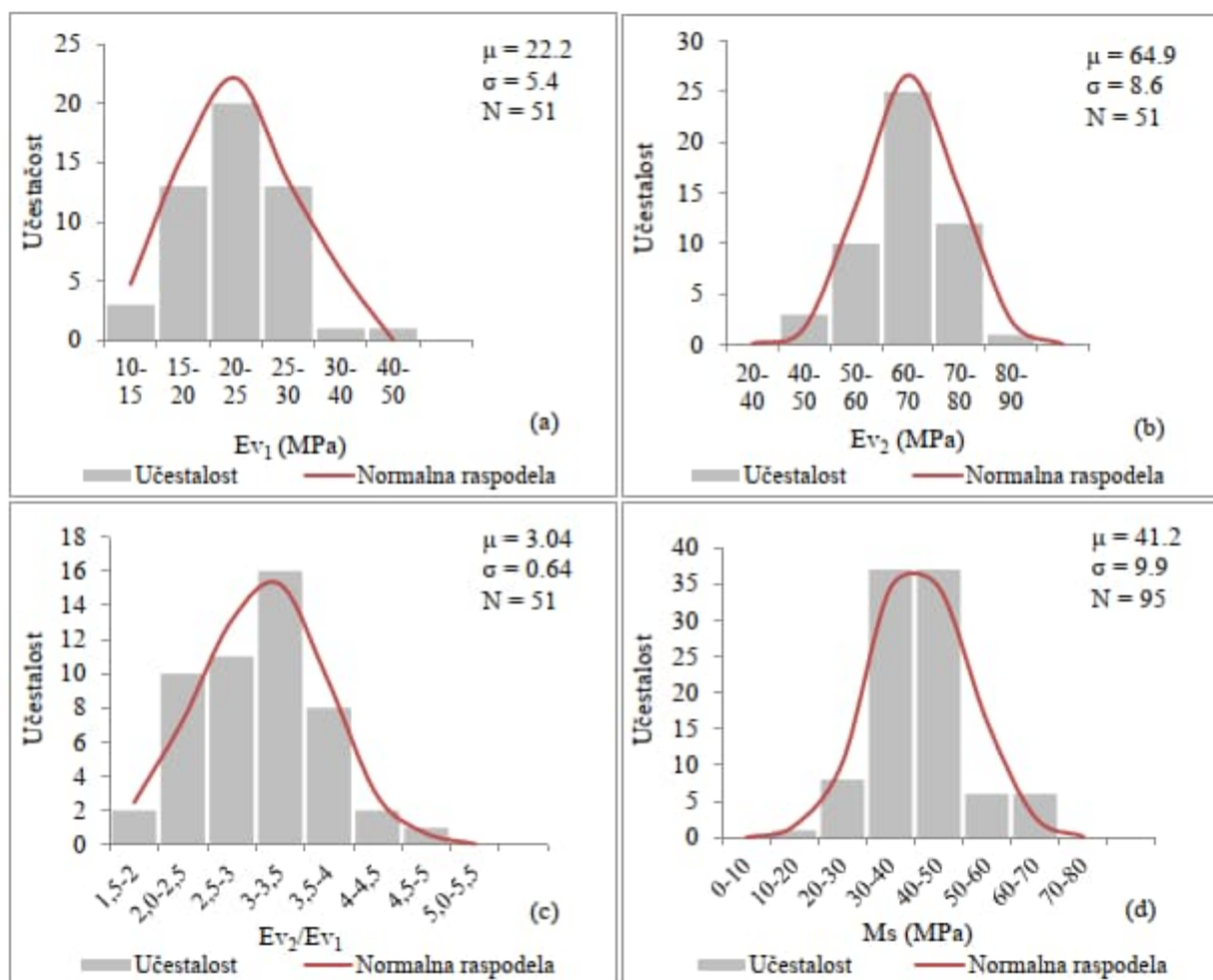
Slika 5.4. Učestalost i distribucija „in situ“ parametara na II sloju nasipa, lokacija L2-S (a) modul deformacije E_{v1} ; (b) modul deformacije E_{v2} ; (c) E_{v2}/E_{v1} ; (d) modul stišljivosti M_s
