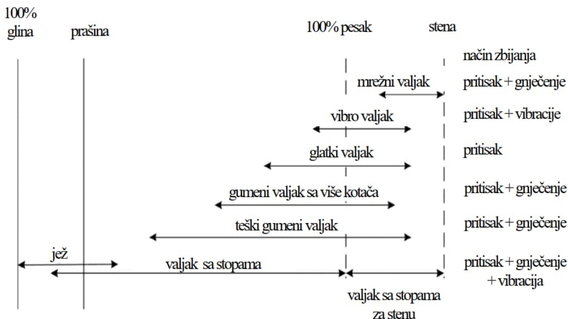
Slika 3.2. Prilagođavanje mehanizacije za zbijanje vrsti materijala (Schroeder, 1975)
