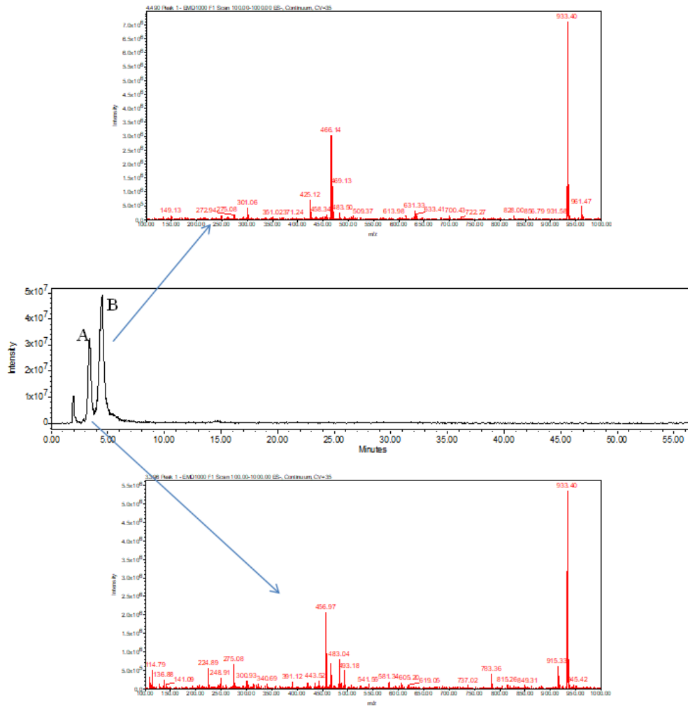
Slika 4.2: Hromatogram veskalagina (A) i kastalagina (B), sa prikazanim spektrima pikova
