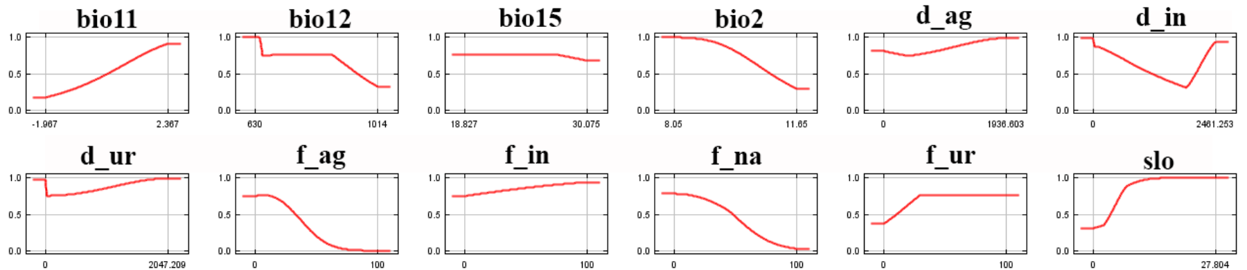
Slika P10.2. Uticaj svih odabranih eko-geografskih varijabli na distribuciju zidnog guštera prema MaxEnt finalnom modelu za region peripanonske Srbije
