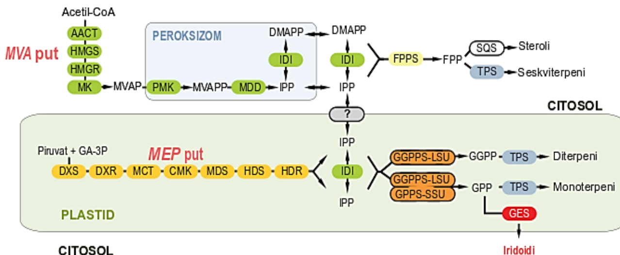
Slika 6. Mreža metaboličkih puteva biosinteze terpena kod biljaka (prema Boachon i sar., 2018). Skraćenice: acetyl-CoA acetyltransferaza (AACT), 3-hidroksi-3-metilglutaril koenzim A sintaza (HMGS); hidroksimetilglutaril-CoA reduktaza (HMGR); ATP:mevalonat-fosfotransferaza (MK); mevalonat 5-fosfat (MVAP); fosfomevalonat kinaza (PMK); mevalonat 5-difosfat (MVAPP); mevalonat difosfat dekarboksilaza (MDD); izopentenil difosfat (IPP); izopentenil difosfat delta-izomeraza (IDI); dimetilalil difosfat (DMAPP); geranil transtransferaza (FPPS); farnezil difosfat (FPP); skvalen sintaza (SQS); terpen sintaza (TPS), 1-deoksi-D-ksilulozo-5-fosfat sintaza (DXS); 1-deoksi-D-ksilulozo-5-fosfat reduktioizomeraza (DXR); 2-C-metil-D-eritritol 4-fosfat, citidilil-transferaza (MCT); 4-(citidin 5-difosfo)-2-C-metil-D-eritritol kinaza (CMK); 2-C-metil-D-eritritol 2,4-ciklodifosfat sintaza (MDS), 4-hidroksi-3-metilbut-2-en-1-il difosfat sintaza (HDS); 1-hidroksi-2-metil-2-(E)-butenil 4-difosfat reduktaza (HDR).
