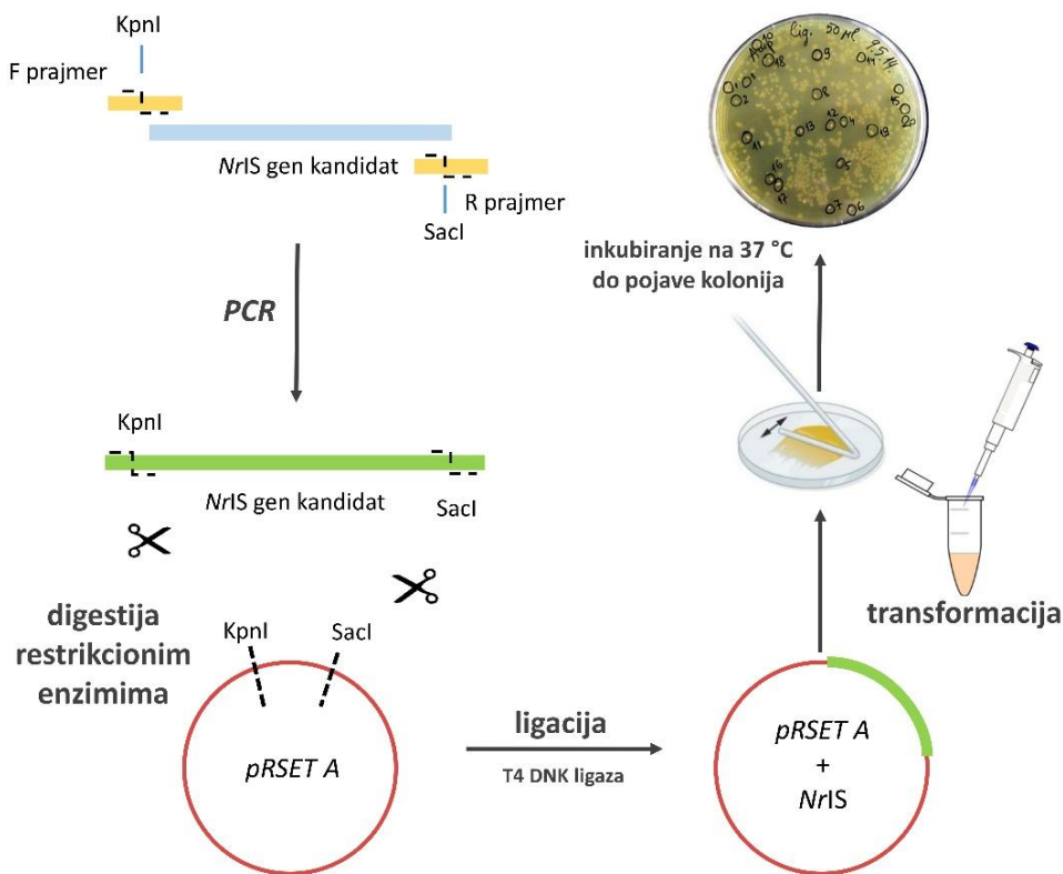
Slika 18. Postupak kloniranja baziranog na restrikcionijskim enzimima na primeru gena kandidata NriS i transformacija kompetentnih ćelija bakterijskih sojeva za ekspresiju ( BL21-CodonPlus (DE3)-RIL i BL21-(DE3)-Rosetta ).
