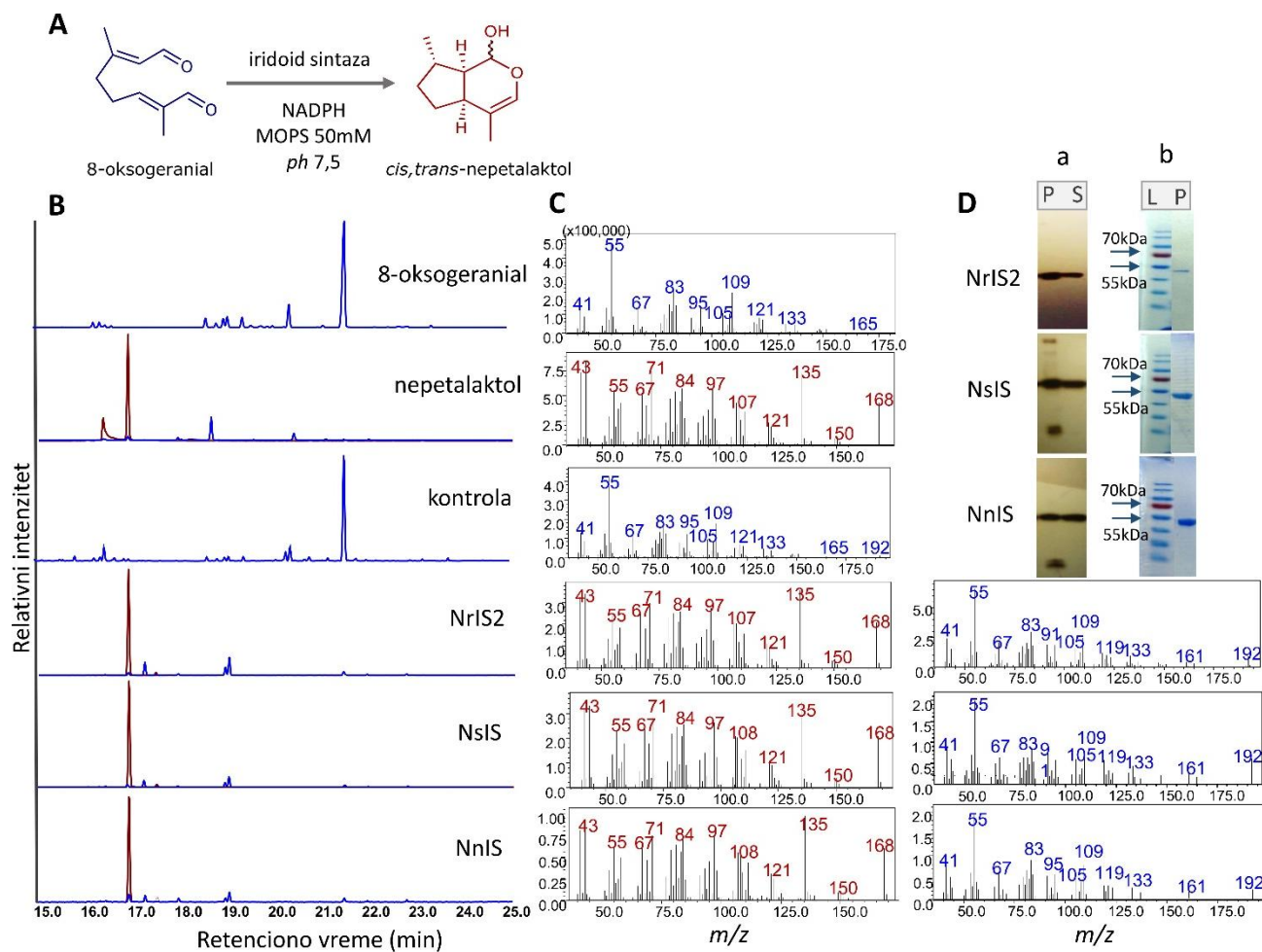
Slika 38. GC-MS analiza enzimskih in vitro esaja sa rekombinantnim enzimima NrIS2, NsIS i NnIS. Prkazana je enzimaska reakcija, u kojoj iridoid sintaza konvertuje 8-oksogeranial do cis,trans -nepetalaktola u puferu sa MOPS koncentracije 50mM i pH 7,5 (A). Upoređeni su ekstrahovani GC-MS hromatogrami za mase 166 i 168 m/z , standarda 8-oksogeraniala i cis,trans -nepetalaktola sa hromatogramima in vitro esaja bez enzima (kontrola) i onih sa rekombinantnim enzimima NrIS2, NsIS i NnIS (B). Retenciono vreme pika koji odgovara nepetalaktolu je R_t=16,9 min, a 8-oksogeranialu R_t=21,5 min. Plavom bojom obeleženi su pikovi koji odgovaraju masama 166 m/z , dok su crvenom bojom obojeni pikovi masa 168 m/z . Na slici su takođe prikazani maseni spektri (C) koji odgovaraju pikovima sa hromatograma levo sa R_t=16,9 min (crveno) i 21,5 min (plavo). Imunoblot (a) i SDS-PAGE (b) pokazuju da su izolovani proteini NrIS2, NsIS i NnIS veličine 42 kDa monomera (D). P – označava uzorak insolubilnih proteina, S – solubilni proteini; L – proteinski marker, P – prečišćeni rekombinantni proteini
