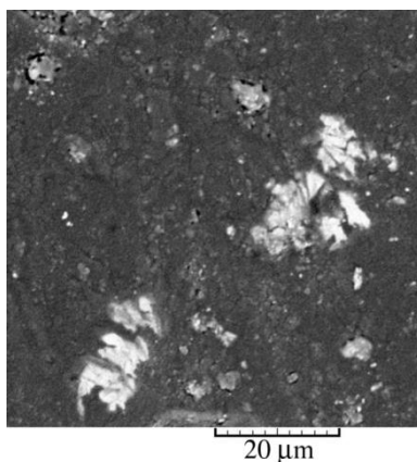
Slika 4.5. SEM slika poprečnog preseka PMMA kompozita ispunjenog galvanostatski proizvedenim bakarnim prahom na perkolacionom pragu. Cu veličina čestica <math>< 45\text{ nm}</math>.
