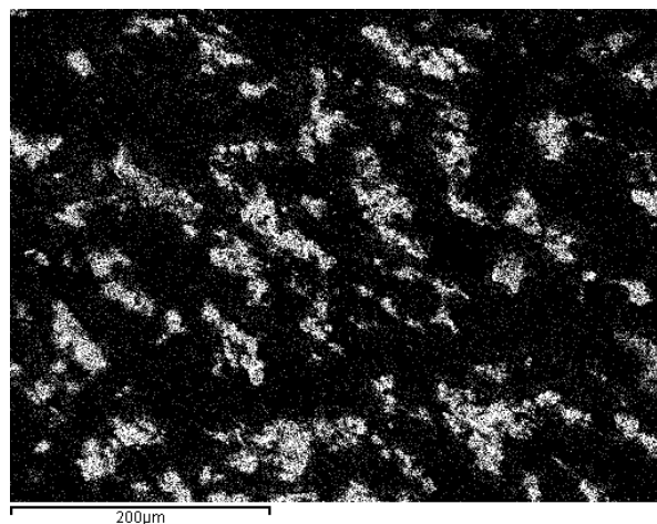
Slika 4.7. EDS slika PMMA kompozita na perkolacionom pragu. Bele tačke predstavljaju Cu prah.
