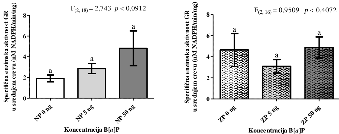
Slika 7. Uticaj benzo[ a ]pirena na specifičnu aktivnost glutation reduktaze u srednjem crevu larvi L. dispar poreklom iz nezagađene šume (nezagađena populacija - NP) i iz zagađene šume (zagađena populacija - ZP), gajenih na veštačkoj dijeti sa dodatkom 0, 5 i 50 ng B[ a ]P po g suve mase hrane. Rezultati su prikazani kao srednja vrednost \pm standardna greška ( \bar{X} \pm SG ). Vrednosti označene različitim slovima razlikuju se značajno ( p < 0,05 ).
