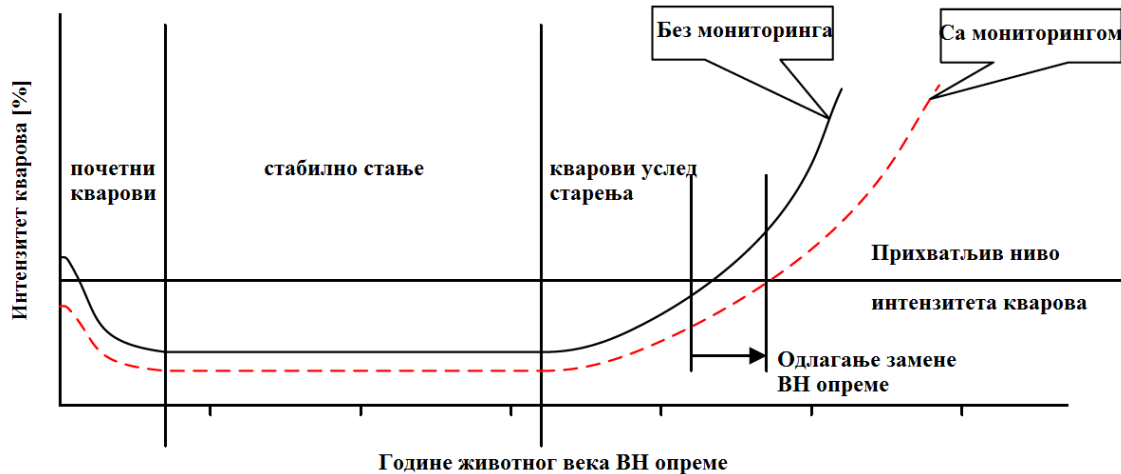
Сл. 2.1.1 Утицај одржавања високонапонске опреме са и без мониторинга на интензитет кварова [1]
