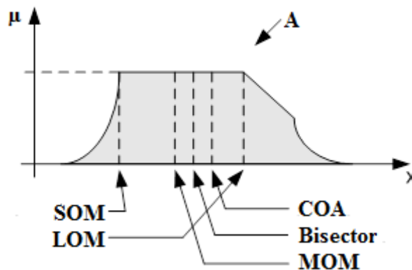
Сл. П1. 0.12 Илустрација метода дефазификације
