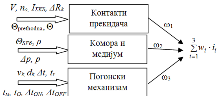
Сл. 3.4.1 Експертски систем прекидача са трима фази експертским подсистемима
