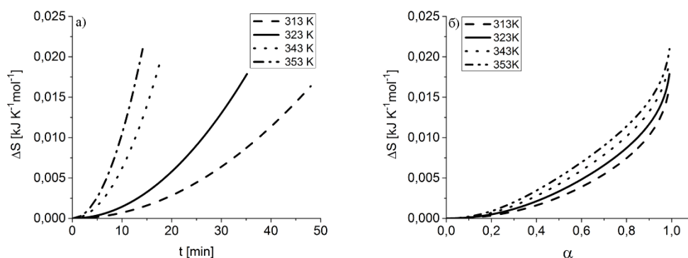
Слика 38. Зависност \Delta S^* изотермне дехидратације PAG хидрогела рачунате по Скрдлином моделу дисперзне кинетике од t (а) и \alpha (б).
