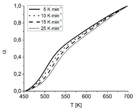
Слика 21. Изотермне ТГ криве дехидратације PAG хидрогела на различитим температурама.
