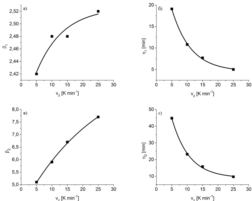
Слика 20. Зависност параметара линеарне комбинације Вејбулових функција ( \beta_1 (а), \eta_1 (б), \beta_2 (в) и \eta_2 (г)) од v_z .
