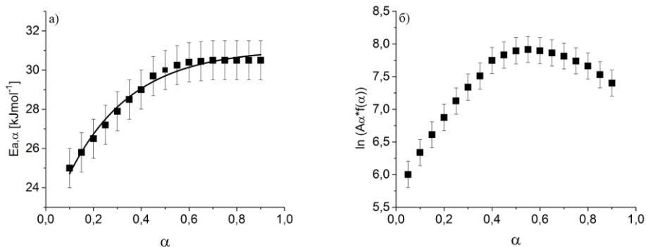
Слика 25. Вредности E_{a,\alpha} (а) и \ln(A_{\alpha}/f(\alpha)) (б) добијене применом интегралног Фридмановог изоконверзионог метода на процес изотермне дехидратације РАГ хидрогела.
