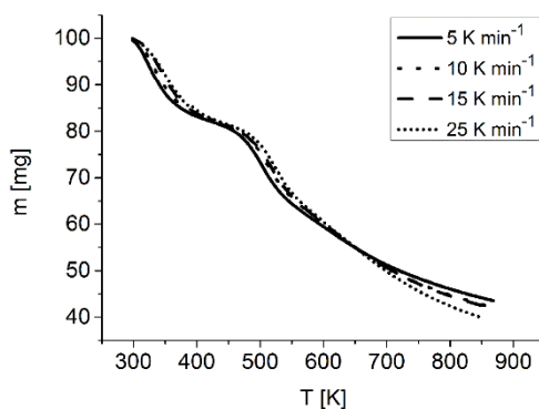
Слика 15. ТГ криве фулерола при различитим брзинама загревања.
