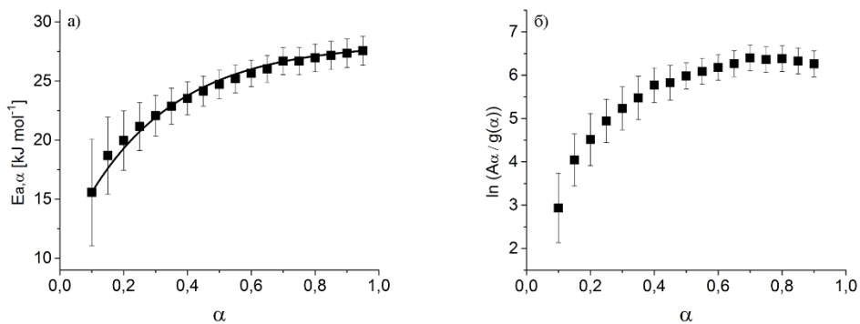
Слика 23. Вредности E_{a,\alpha} (а) и \ln(A_{\alpha} * f(\alpha)) (б) добијене применом диференцијалног Фридмановог изоконверзионог метода на процес изотермне дехидратације PAG хидрогела.
