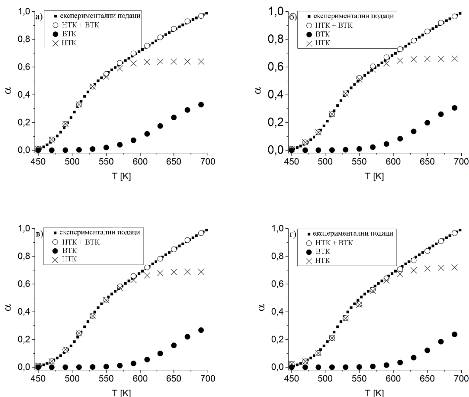
Слика 19. Резултати описивања неизотермене дехидроксилације фулерила линеарном комбинацијом двеју Вејбулових функција и компоненте линеарне комбинације за различите v_z : а) 5 K min -1 , б) 10 K min -1 , в) 15 K min -1 и г) 25 K min -1 . (НТК-нискотемпературска компонента, ВТК-високотемпературска компонента)
