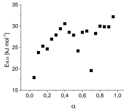
Слика 27. Вредности E_{a,\alpha} добијене применом Вјазовкиновог изоконверзионог метода на процес изотермне дехидратације РАГ хидрогела.
