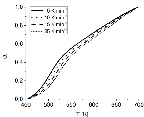
Слика 16. Зависност \alpha од T за реакцију дехидроксијације фулерола на различитим v_z .
