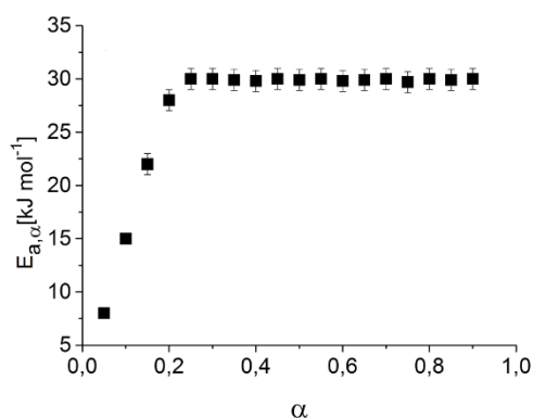
Слика 33. Вредности E_{a,\alpha} добијене применом диференцијалног Фридмановог изоконверзионог метода на процес изотермног испаравања воде.
