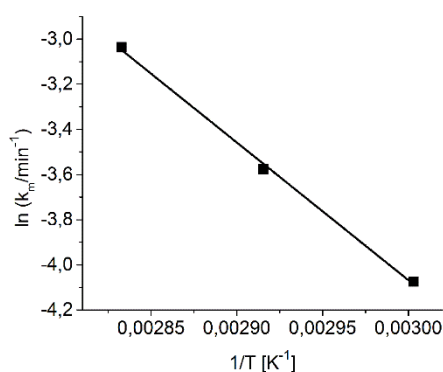
Слика 42. График зависности \ln(k_m / \text{min}^{-1}) од 1/T за процес изотермне дехидратације РАГ хидрогела у условима микроталасног загревањем са константним хлађењем.
