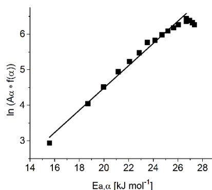
Слика 26. Компензациона релација између привидних кинетичких параметара изотермне дехидратације PAG хидрогела добијених интегралним Фридмановим изоконверзионим методом.
