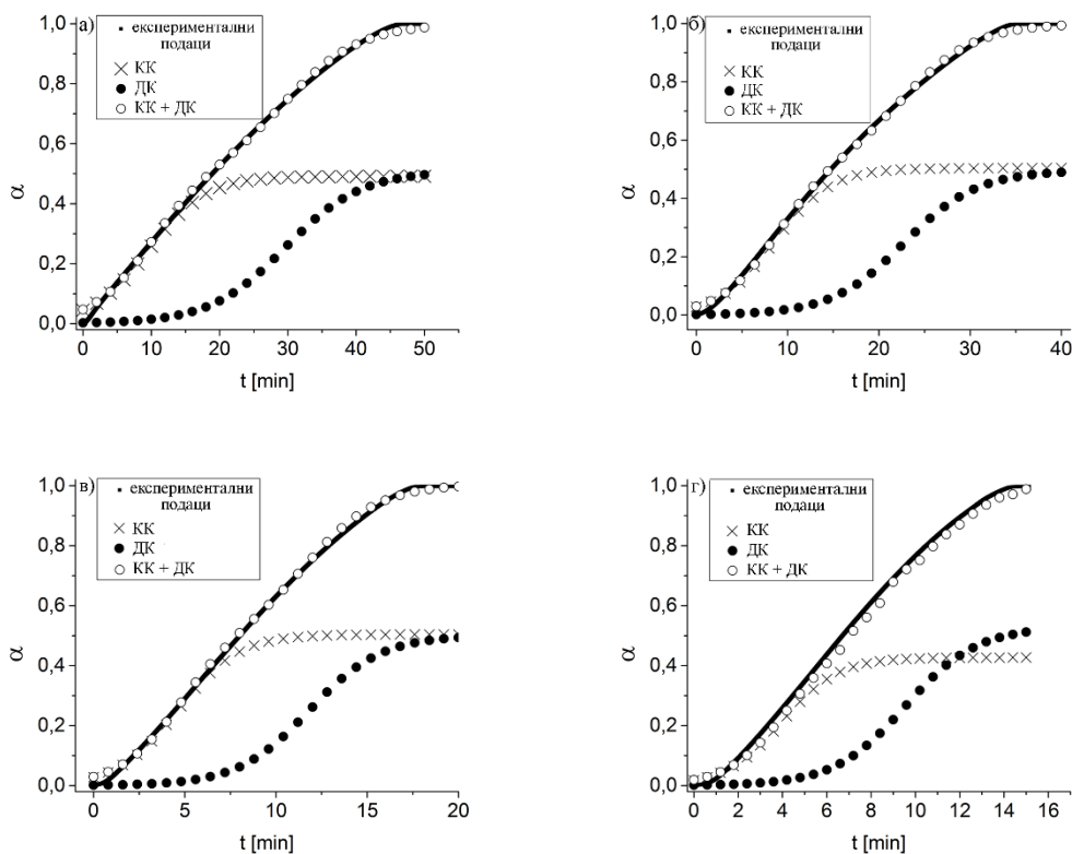
Слика 29. Резултати описивања изотермне дехидратације PAA хидрогела линеарном комбинацијом двеју логистичких функција и компоненте линеарне комбинације на различитим температурама: а) 313К, б) 323К, в) 343К и г) 353К.
