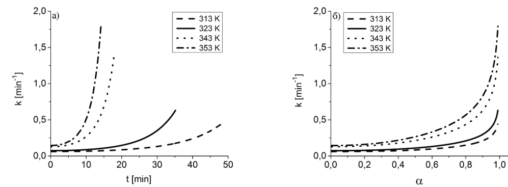
Слика 36. Зависност k изотермне дехидратације PAG хидрогела рачунате по Скрдлином моделу дисперзне кинетике од t (а) и \alpha (б).
