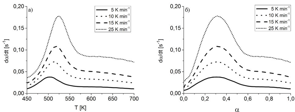
Слика 17. Зависност da/dt од T (а) и \alpha (б) за реакцију неизотермне дехидроксилације фулерола.
