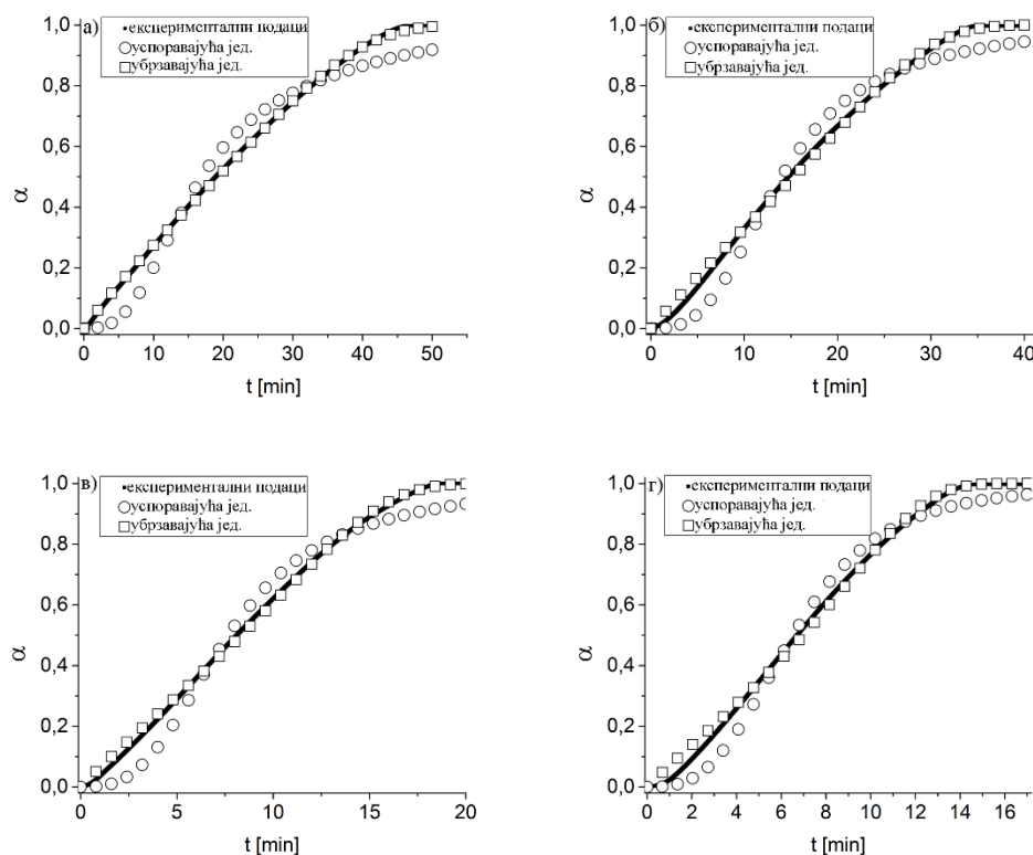
Слика 34. Резултати описивања изотермне дехидратације PAA хидрогела успоравајућом и убрзавајућом моделном једначином Скрдлиног модела дисперзне кинетике на различитим температурама: а) 313К, б) 323К, в) 343К и г) 353К.
