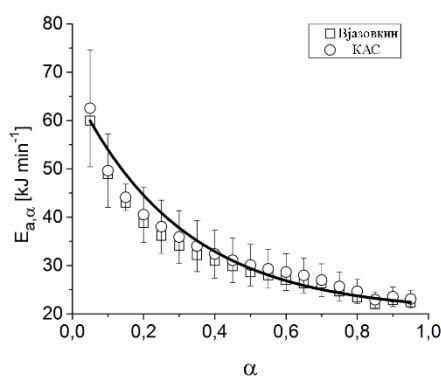
Слика 7. Вредности E_{a,\alpha} добијене Вјазовкиновим и КАС изоконверзионим методом за процес неизотермне дехидратације РАГ хидрогела.
