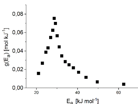
Слика 9. Функција расподеле енергија активације за процес изотермне дехидратације PAG хидрогела
