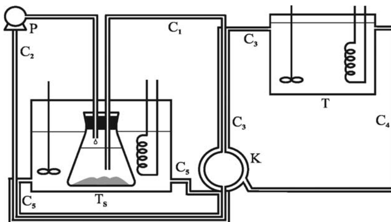
Slika 24. Eksperimentalni uređaj
