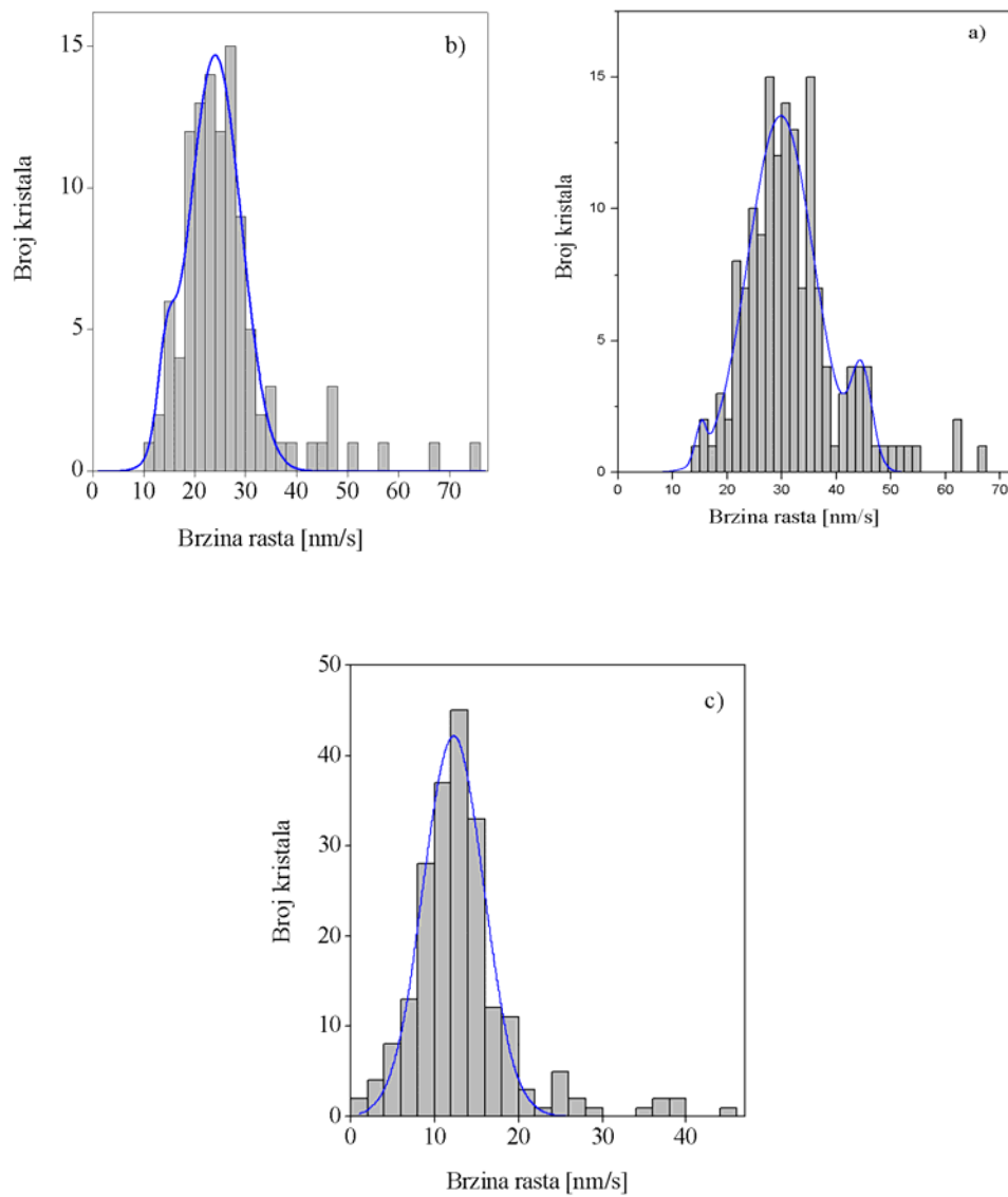
Slika 34. Histogrami predstavljaju raspodelu brzina rasta KDP kristala: a) u \langle 100 \rangle pravcu pre rastvaranja, b) u \langle 100 \rangle pravcu posle refacetiranja i c) \{100\} plosni posle refacetiranja [130]
