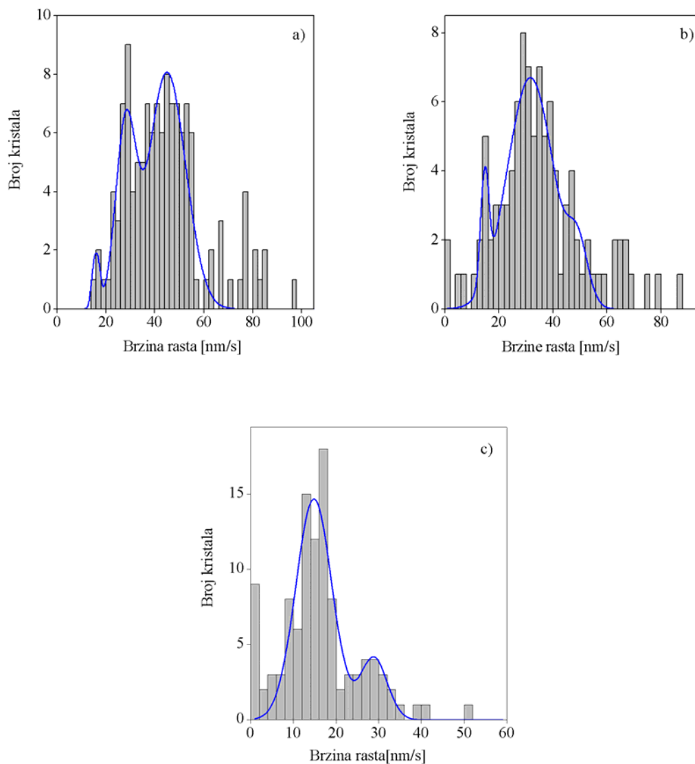
Slika 35. Histogrami brzina rasta KDP kristala: a) u [001] pravcu pre rastvaranja, b) u [001] pravcu posle refacetiranja i c) krovova posle refacetiranja [130]
