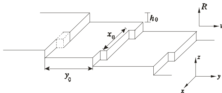
Slika 10. Stepenci sa označenim karakterističnim veličinama
