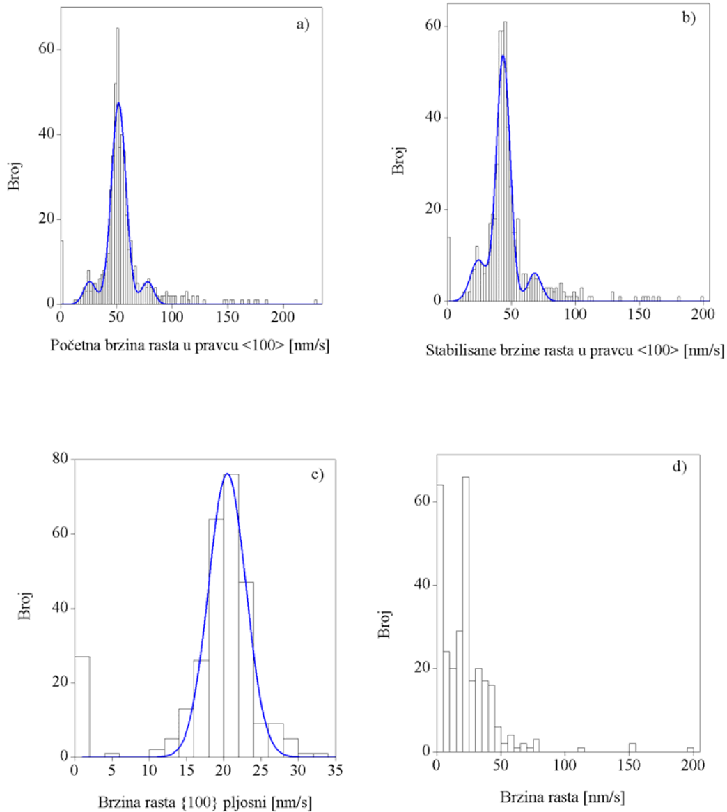
Slika 31. Histogrami disperzije: a) početnih brzina rasta, b) stabilisanih brzina rasta, c) srednjih brzina rasta posle refacetiranja, d) srednjih brzina rasta kristala u eksperimentima druge serije [198].
