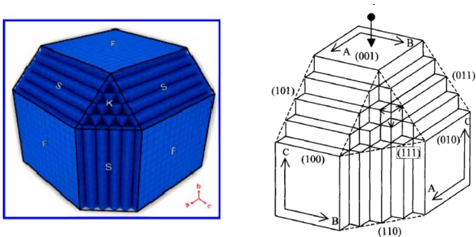
Slika 8: F , S i K pljosni kristala sa tri lanca periodičnih veza (pravci su naznačeni crvenom bojom na slici levo) [31]
