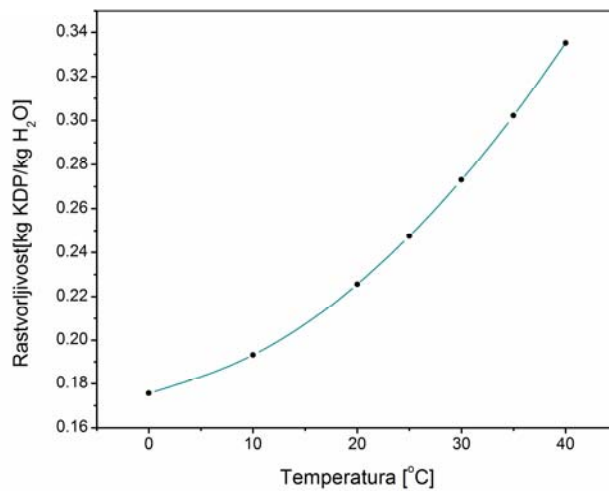
Slika 22. Rastvorljivost kalijum dihidrogen fosfata
