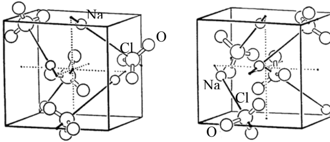
Slika 20. Atomsko uređenje natrijum hlorata [23]
