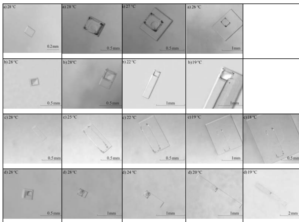
Slika 32. Primeri vremenske evolucije četiri kristala (označeni sa a, b, c i d). U prvoj koloni su slike kristala na 28°C pre rastvaranja, a u ostalim slike kristala na različitim temperaturama posle refacetiranja.
