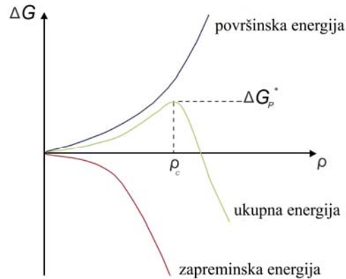
Slika 9. Zavisnost energije nukleacije od radijusa nukleusa
