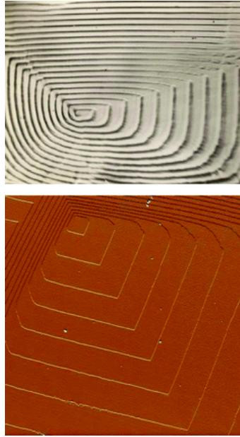
Slika 15. Spiralni makrostepenik saharoze [76] i kalijum hidrogen ftalata [83].
