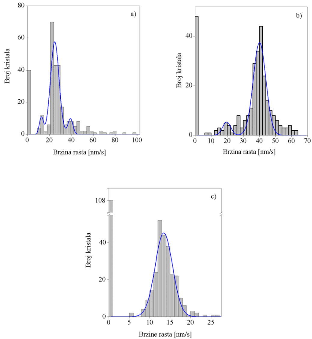
Slika 33. Histogrami raspodele brzina rasta kristala natrijum hlorata: a) u \langle 100 \rangle pravcu pre rastvaranja, b) u \langle 100 \rangle pravcu posle rastvaranja, c) plosni \{100\} posle refacetiranja [130]
