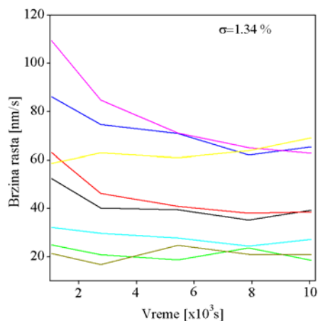
Slika 29. Vremenska evolucija brzina rasta pre rastvaranja
