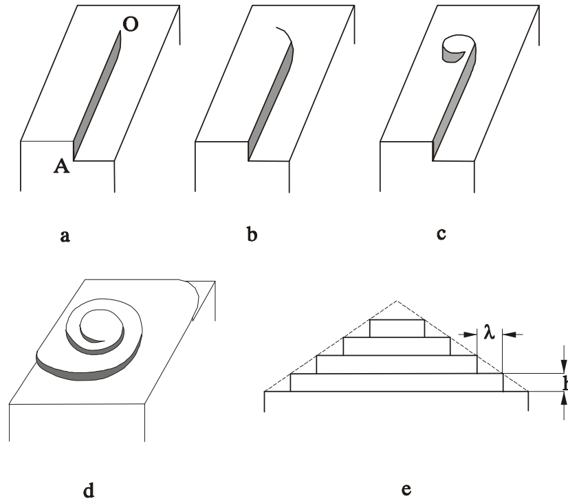
Slika 13. Nastajanje dislokacionog brežuljka oko dislokacione tačke [23]
