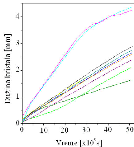
Slika 28. Zavisnost dužine kristala u određenom pravcu od vremena
