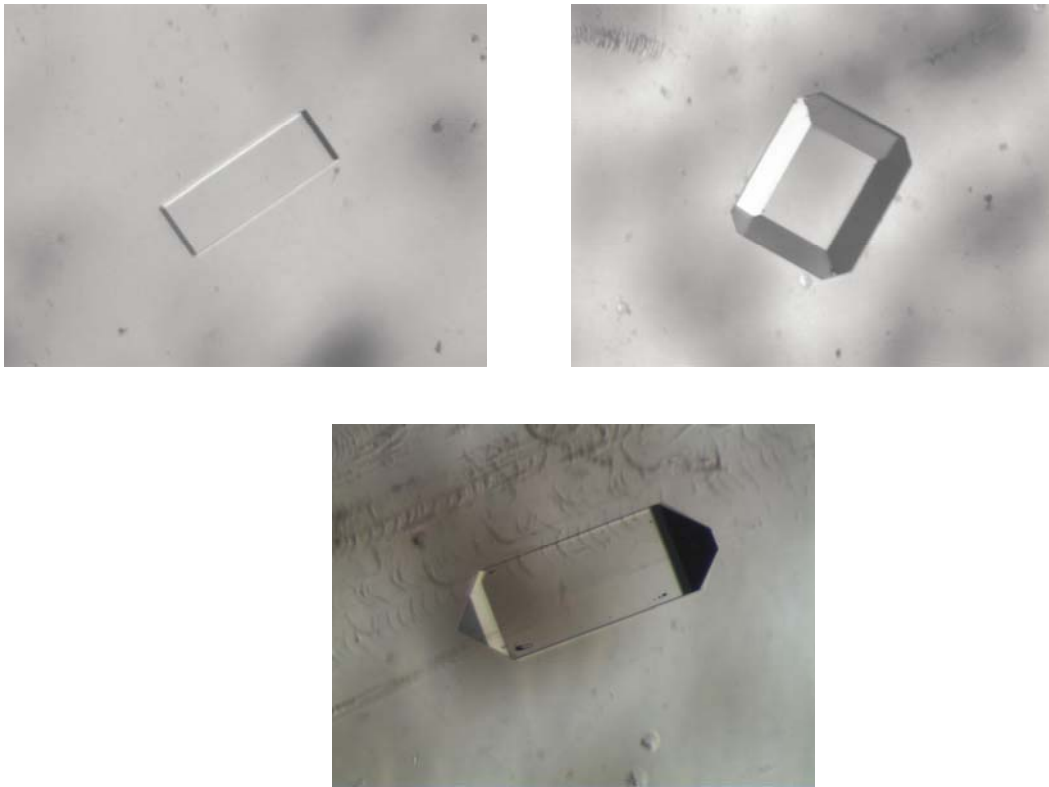
Slika 27. a) i b) kristal natrijum hlorata sa i bez pljosni viših indeksa c) izgled KDP kristala
