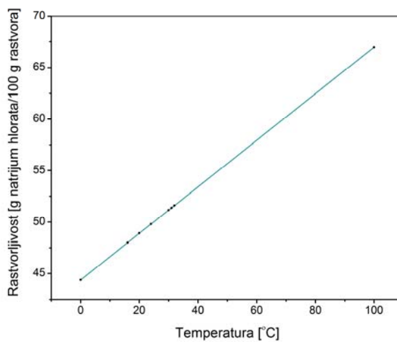
Slika 23. Rastvorljivost natrijum hlorata
