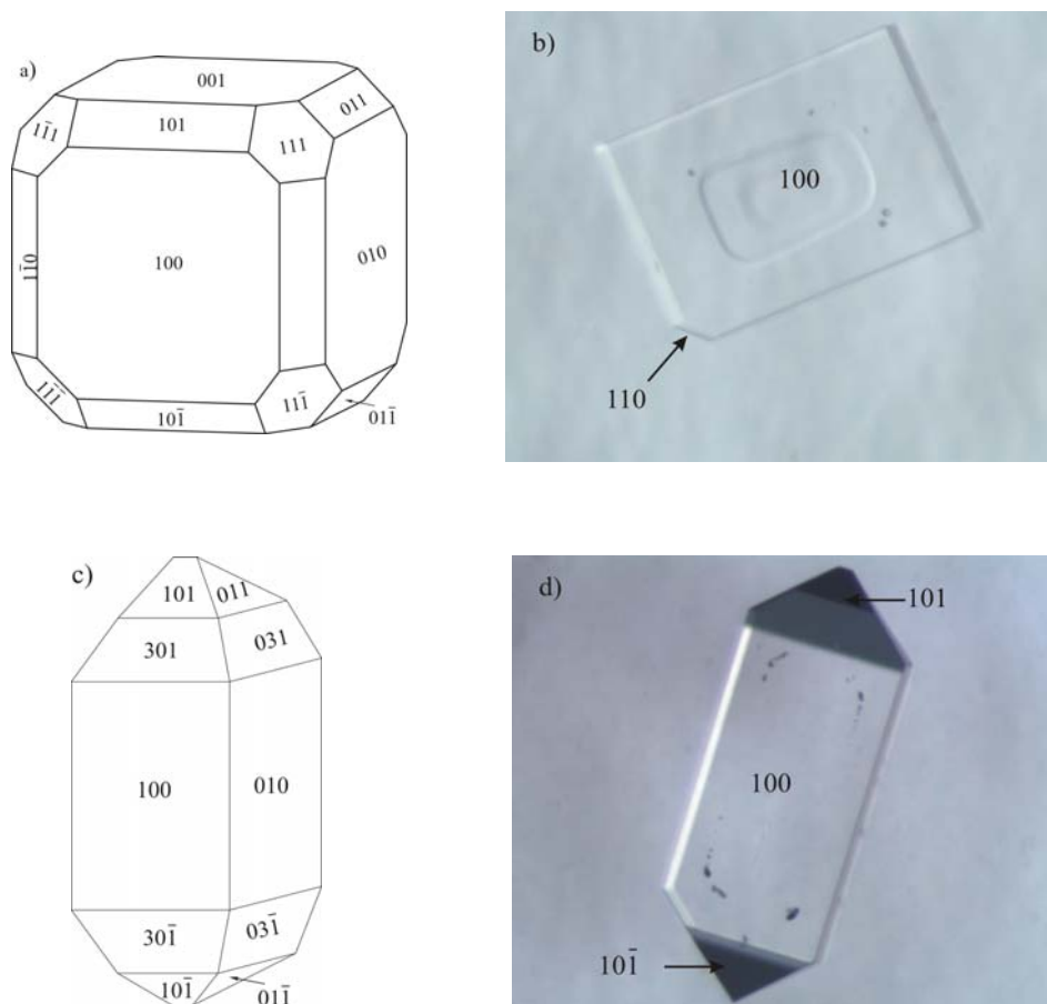
Slika 26. a) Šematski i b) eksperimentalno posmatran habitus kristala natrijum hlorata, i c) šematski i d) eksperimentalno posmatran habitus kristala KDP-a [130]
