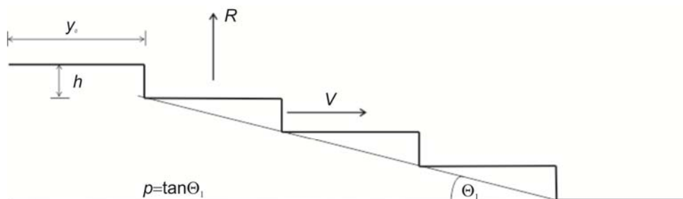
Slika 17. Niz stepenika koji formiraju spiralni brežuljak
