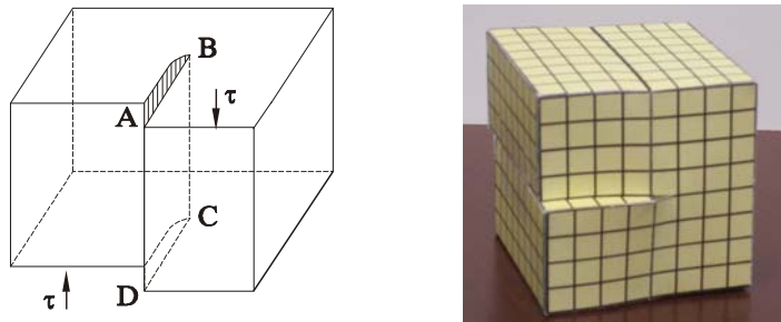
Slika 12. Nastanak zavojne dislokacije
