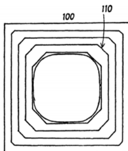
Slika 21. Iščezavanje pljosni viših indeksa prilikom rasta posle rastvaranja
