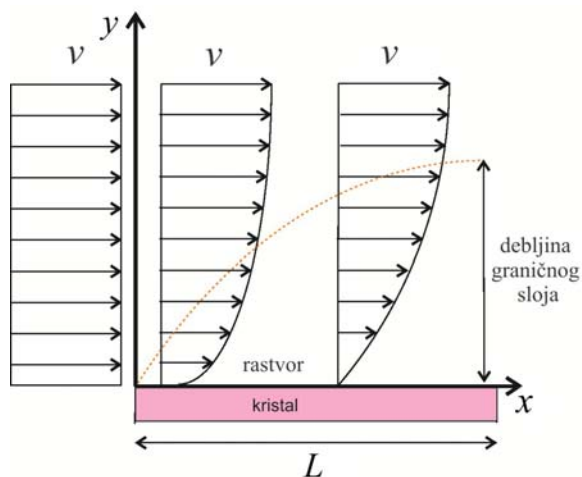
Slika 1. Zavisnost brzine rastvora od udaljenosti od pljosni kristala.
