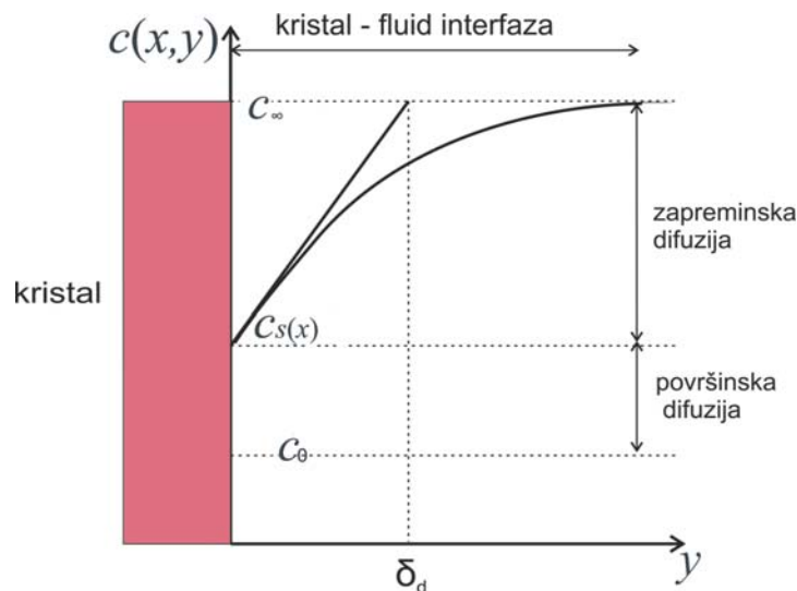
Slika 3. Zavisnost koncentracije rastvora od normalne udaljenosti od pljosni kristala y , na fiksnoj udaljenosti od čone ivice x
