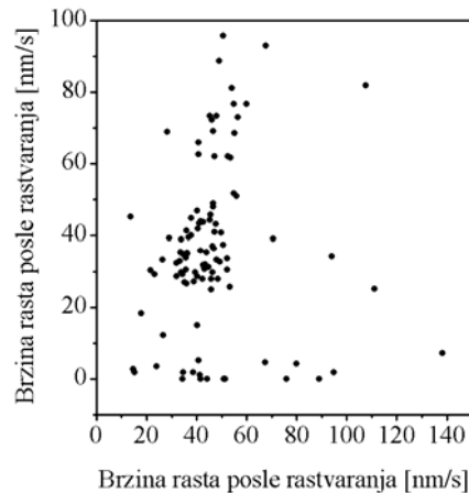
Slika 30. Korelacija između brzina rasta posle rastvaranja i brzina rasta pre rastvaranja [198]
