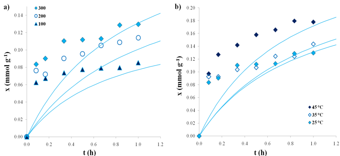
Slika 4.9 Eksperimentalni podaci (simboli) i predviđanja modela kinetike pseudo-drugog reda (linije) u toku prvih sat vremena: a) iz rastvora sa početnim koncentracijama 100 – 300 \text{mgCu dm}^{-3} na 25 °C; b) iz rastvora sa početnom koncentracijom 300 \text{mgCu dm}^{-3} na 25 – 45 °C (eksperimentalni podaci su srednje vrednosti dva merenja; standardne devijacije eksperimentalnih podataka su izostavljane radi preglednosti)
