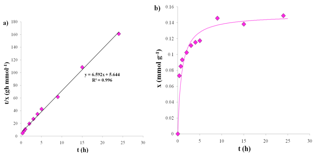
Slika 4.15 Primena modela kinetike pseudo-drugog reda na eksperimentalne podatke (simboli) za početnu koncentraciju 300 \text{ mgMn dm}^{-3} na 25 \text{ }^\circ\text{C} : a) primena modela u linearizovanom obliku; b) koncentracija Mn(II) na zeolitu tokom 24 h: eksperimentalni podaci (srednje vrednosti dva merenja; simboli) i predviđanja modela (linija), (standardne devijacije eksperimentalnih podataka su izostavljane radi preglednosti)
