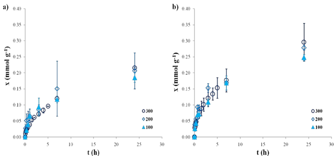
Slika 4.35 Koncentracija Cu(II) na zeolitu A, x , u zavisnosti od vremena za C_0 = 100, 200 i 300 \text{ mgCu dm}^{-3} na 20 \text{ }^\circ\text{C} : a) velike kuglice; b) male kuglice (eksperimentalni podaci su srednje vrednosti dva merenja)
