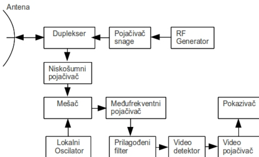
Slika 1.4: Blok šema podsistema koji se mogu naći u radaru.
