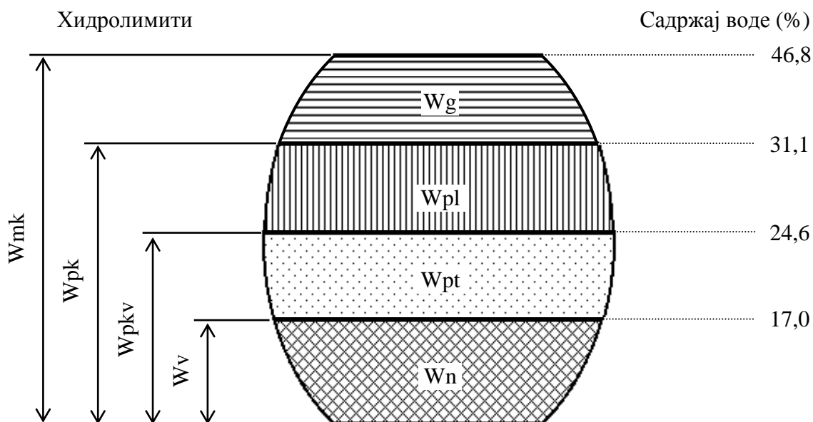
Сл. 2. Хидролимити чернозема и приступачност воде у ефективној дубини ризосфере кукуруза (хидролимити: W_v – винућа, W_{pkv} - прекида капиларне везе, W_{pk} - пољског капацитета и W_{mk} - максималног капацитета)
