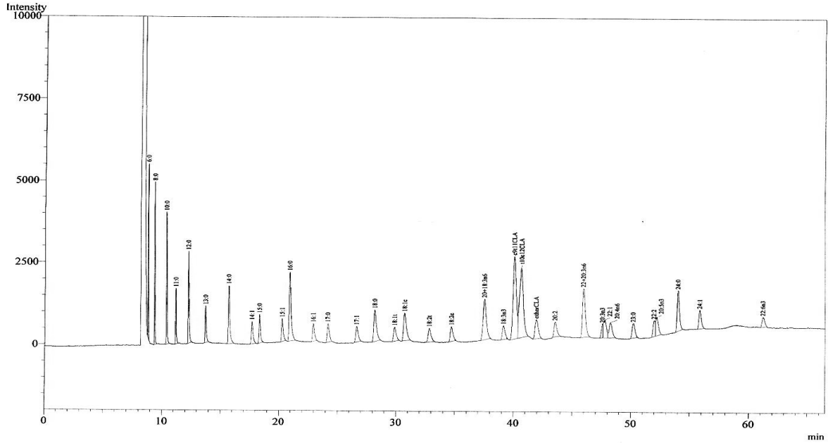
Slika 4.3. GC hromatogram metilestara masnih kiselina u smeši standardnog rastvora Supelco 37 Component FAME Mix i smeše izomera metilestara cis -9 trans -11 trans -10 cis -12-oktadekadienske kiseline
