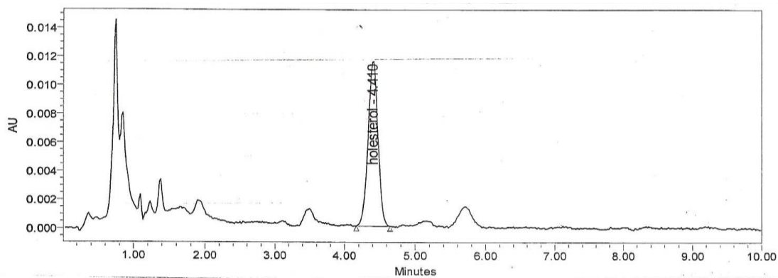
Slika 4.7. Hromatogram standardnog rastvora holesterola koncentracije 25 mg/L u acetonitril/izopropanolu (20% / 80%, v/v)
