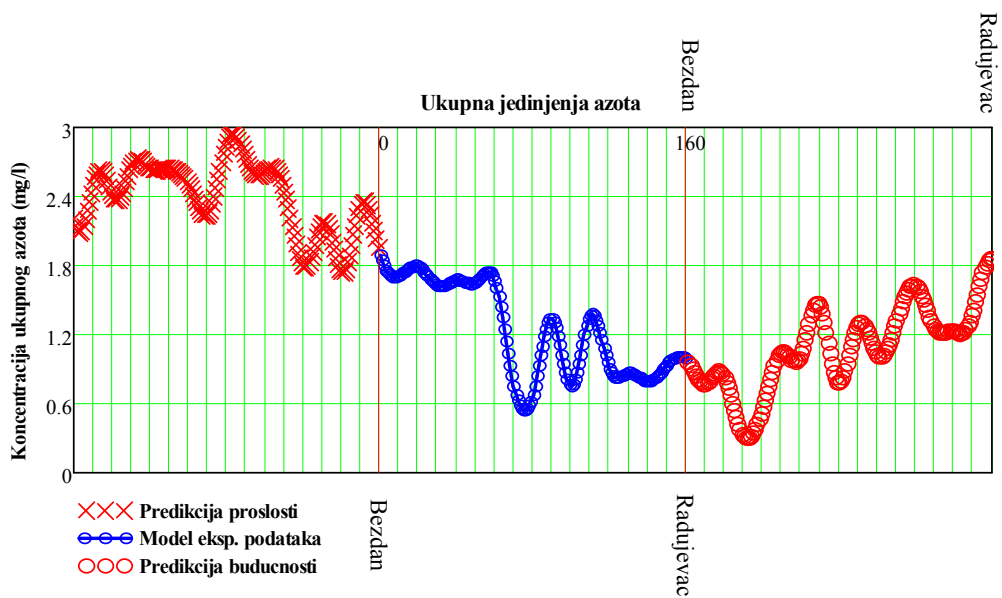
Slika 6.31. Dinamika koncentracije ukupnih jedinjenja azota u 2009. godini, i krive predviđanja budućih i prošlih stanja u vodotoku
