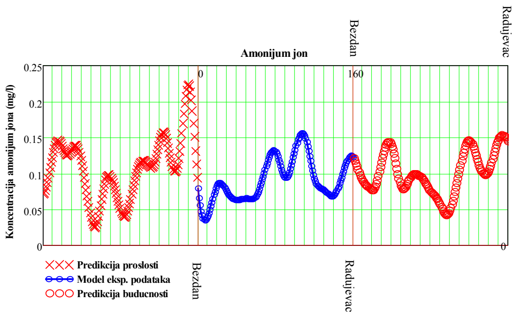
Slika 6.32. Dinamika koncentracije ukupnih amonijumovih jona u 2009. godini i krive predviđanja budućih i prošlih stanja u vodotoku
