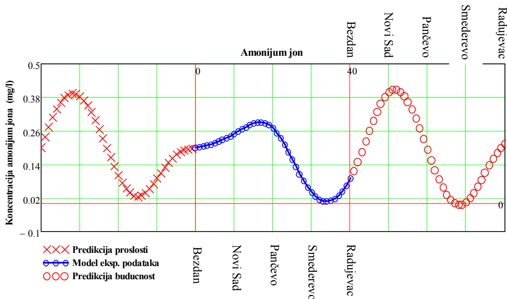
Slika 6.30. Krive predviđanja budućih i prošlih stanja koncentracije amonijum jona u vodotoku u odnosu na 2006. godinu
