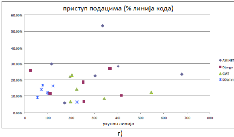
Слика 51. Поређење различитих аспеката анализираних апликација. Процент линија програмског кода потрошен на дефинисање а) графичких елемената у модулу, б) распореда, в) понашања и г) приступа подацима.
