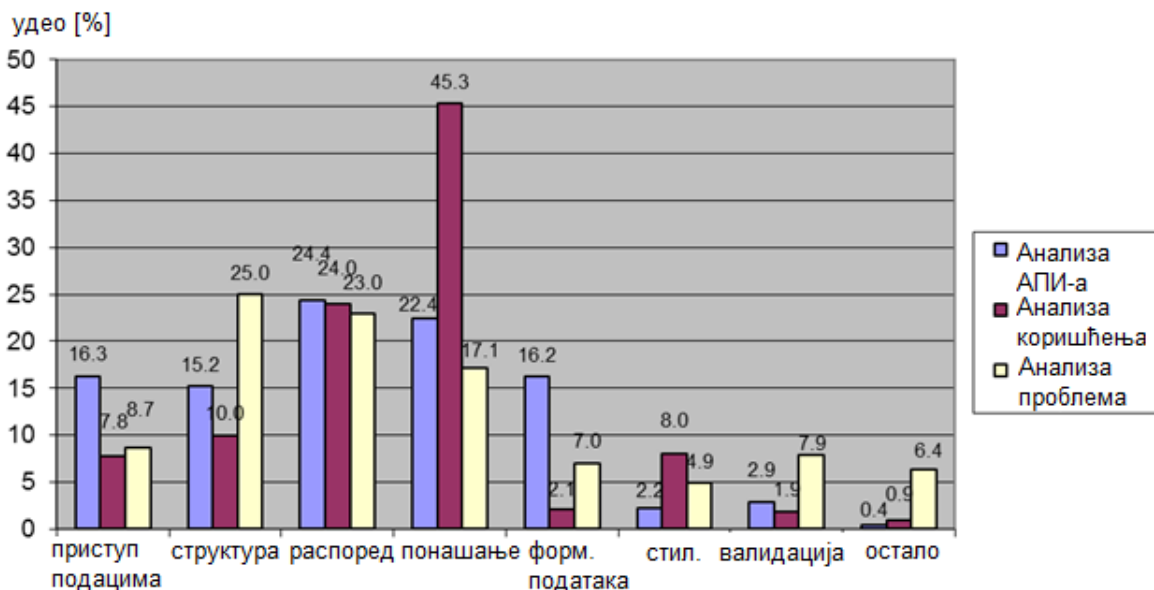
Слика 3. Резултати анализе апликативног програмског интерфејса, анализе коришћења елемената истог интерфејса и анализе проблема из репозиторијума.
