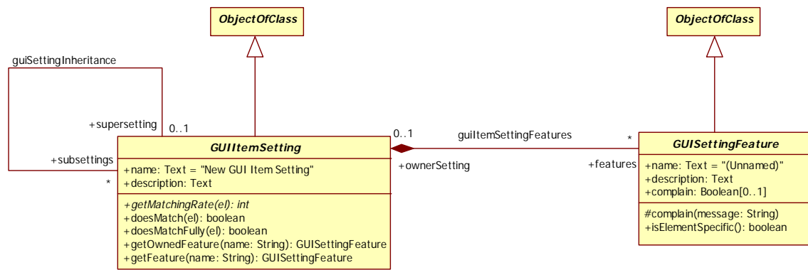
Слика 22. Модел пакета за форматирање података на језику UML.
