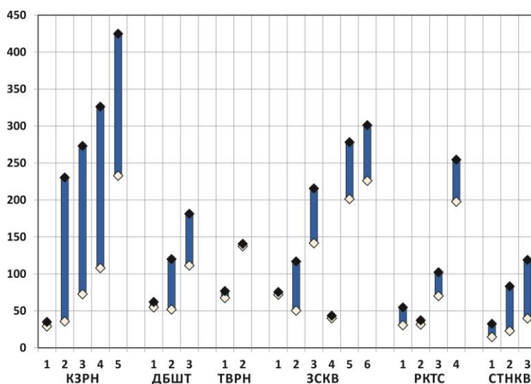
Слика 5.2.30. Промена средње годишње запремине укупних количина вученог и суспендованог наноса G_{god} на истраживаним подсливовима (стање пре и након уноса туристичко-рекреативних елемената)
