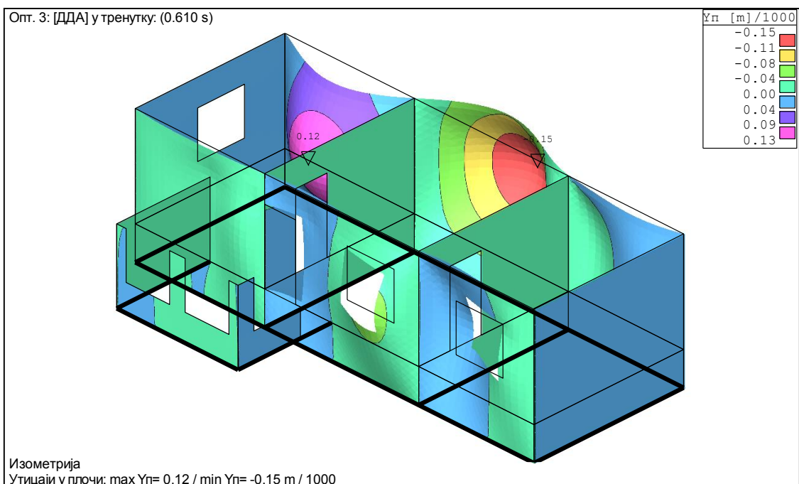
Слика 39: Померања у Y правцу
