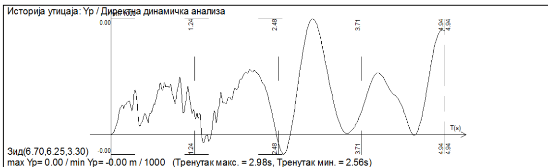
Слика 29: Анализа померања у зиду, који показује највећа померања у У правцу (подужни зид, који је пре доградње ветробрана био улазни фасадни зид)
