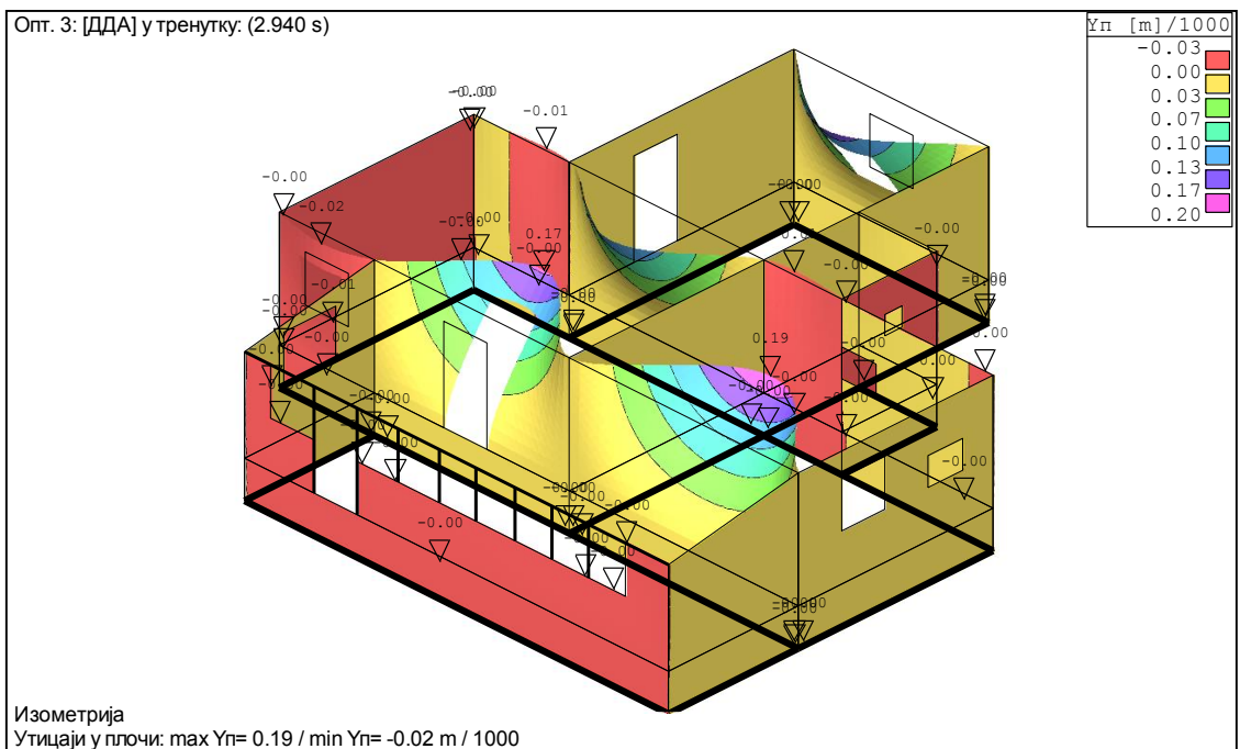
Слика 31: Померања у Y правцу
