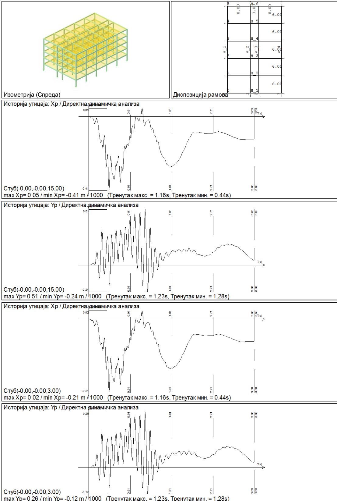
Слика 87: П+4: 3д модел, основа, максимална укупна и релативна померања.
