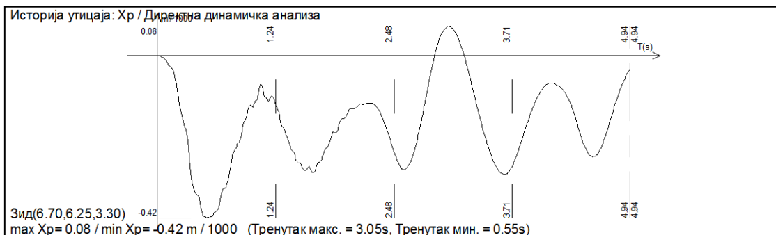
Слика 28: Анализа померања у зиду који показује највећа померања у Х правцу (средњи попречни зид)
