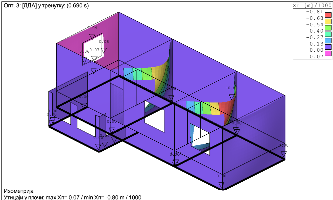
Слика 38: Померања у X правцу
