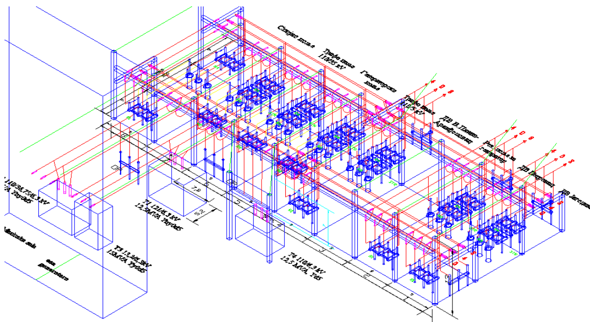
Slika 7.27: 3D prikaz 110 kV postrojenja TE "Morava"
