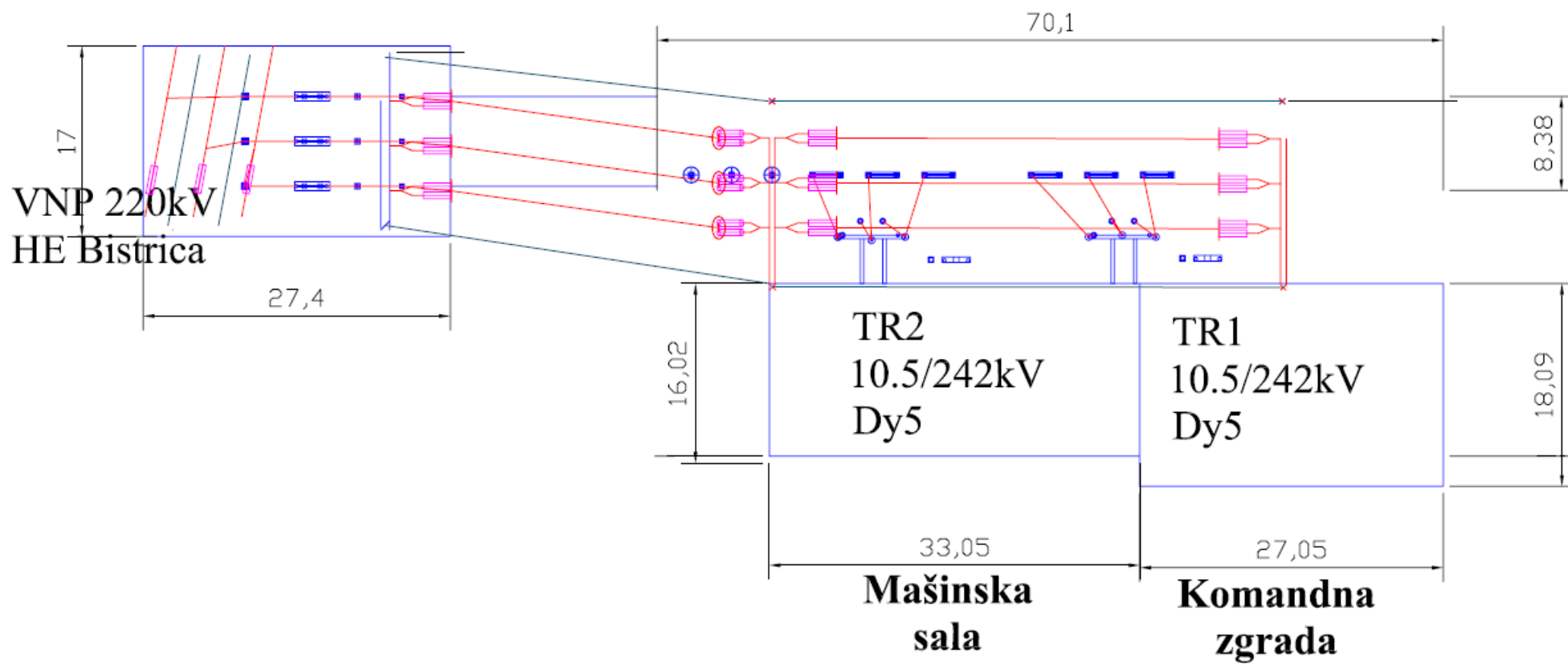
Slika 10.21: 2D prikaz dispozicije 220 kV postrojenja HE "Bistrica"
