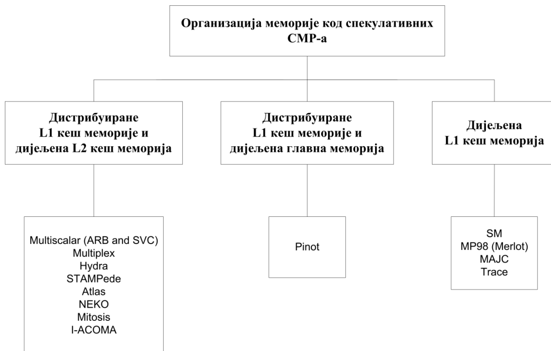
Слика 4-1. Класификација спекулативних CMP-ова са подршком за меморијску комуникацију између спекулативних нити
