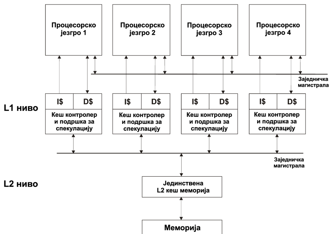
Слика 5-1. Структура предложеног система
