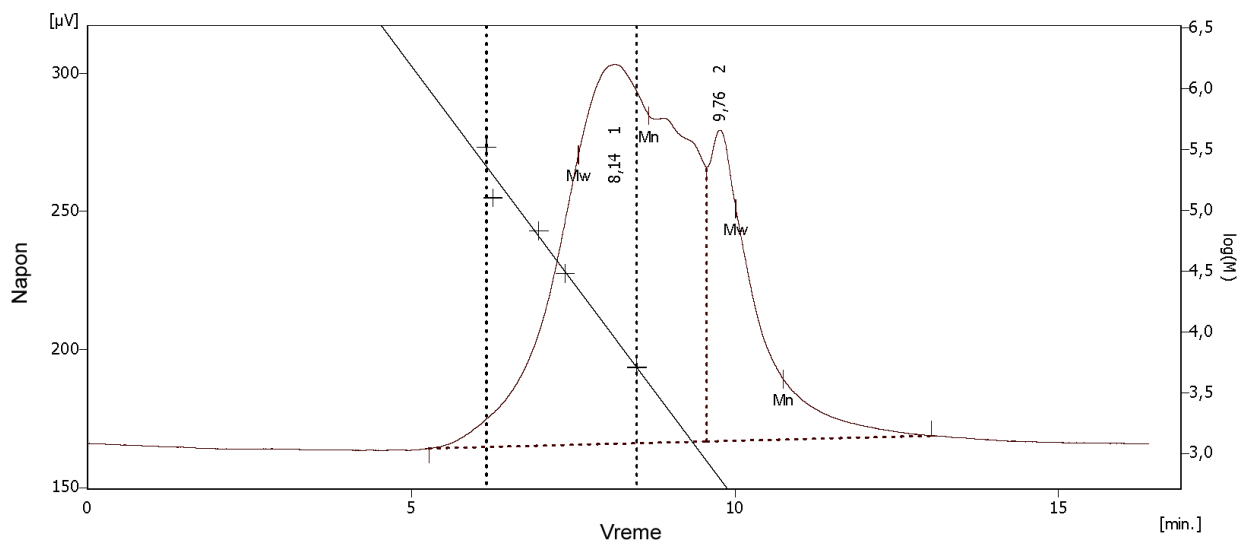
Slika 41. Hromatogram za uzorak PANI-0.05: Prikaz signala detektora/ \log(M) u funkciji od retencionog vremena.
