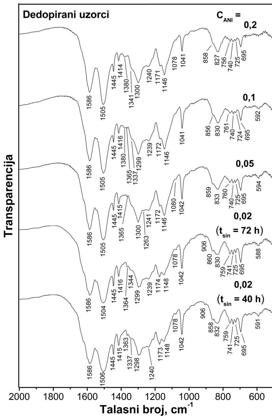
Slika 48. Normirani FTIR spektri dedopiranih uzoraka PANI-0.02-40-dedop, PANI-0.02-72-dedop, PANI-0.05-dedop, PANI-0.1-dedop i PANI-0.2-dedop u spektralnoj oblasti 2000\text{--}500 \text{ cm}^{-1} . Vrednosti C_{\text{ANI}} označene su uz odgovarajući spektar.
