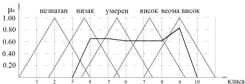
Слика број 5.23 Фази скуп ризика отказа за главну хидропумпу
