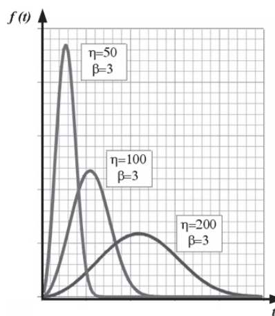
Слика број 2.5 Понашање Вејбулове расподеле релативних фреквенци f(t) у зависности од вредности параметра паразмере \eta ( www.weibull.com )
