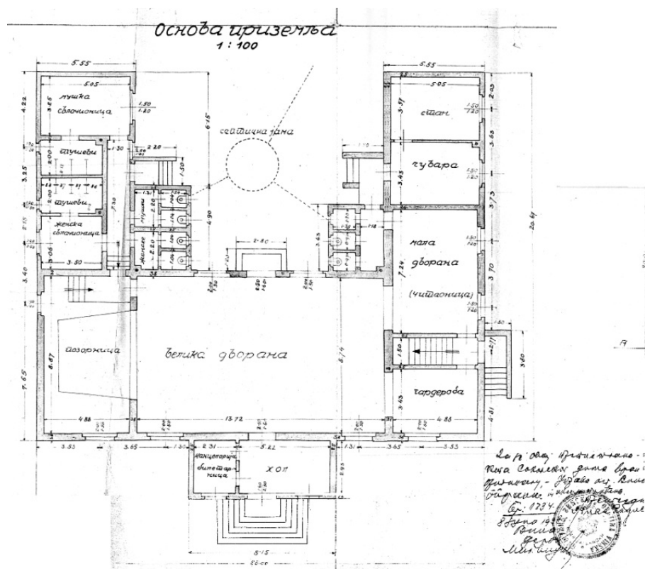
Слика 74 - Пројекат Соколског дома у Вини, основа приземља, 1937. (АЈ, Фонд МФВ)
