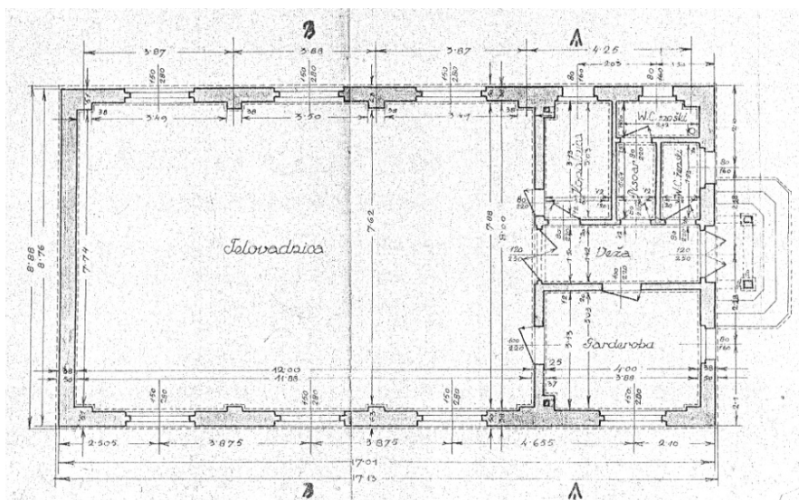
Слика 127 - Пројекат Соколског дома у Марковцима, основа приземља, 1938. (АЈ, Фонд МФВ)
