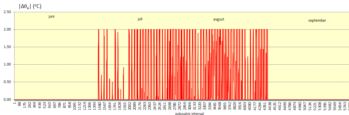
Slika VII.20 Sniženja temperature prostorijâ usled dodatnog angažovanja klima uređaja, po varijanti 2 modela DSM (odgovarajuća slučaju sa slike VII.19)
