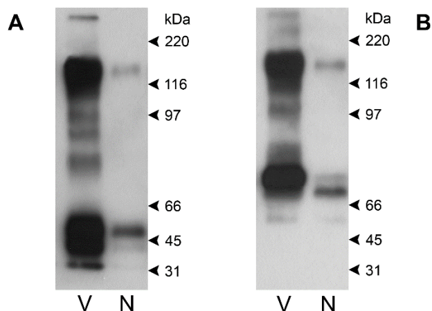
Slika 10. Imunoblot vezane (V) i nevezane (N) frakcije posle IMAC koristeći matriks sa imobilizovanim \text{Fe}^{3+} jonima. Imunoreaktivni proteini su prepoznati u interakciji sa anti-IGFBP-3 ( A ), odnosno anti-Tf antitelima ( B ).
