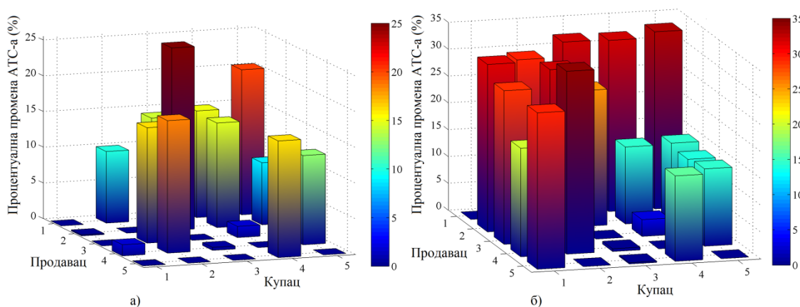
Слика 5.12. а) Проценат промене вредности АТС-а када су уважавана само напонска ограничења, б) Проценат промене вредности АТС-а када су уважавана сва релевантна ограничења.
