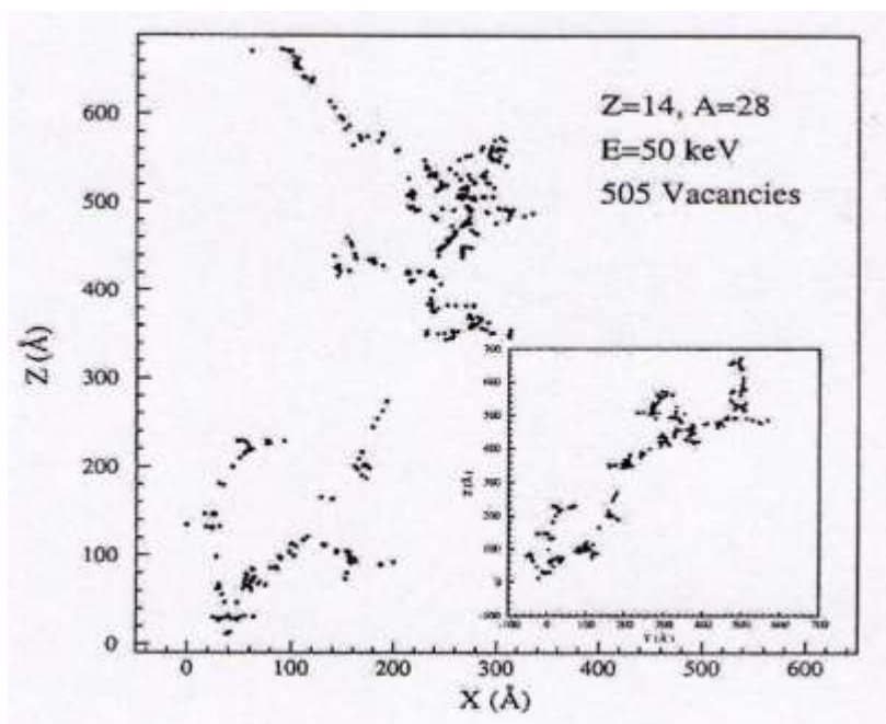
Slika 25. Prostorna raspodela vakanacija pri upadnoj energiji od 50keV. Mala slika pokazuje poprečnu projekciju istog događaja. [38]
