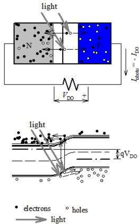
Slika 10. Solarna ćelija: a) poprečni presek, b) dijagram energetske zone pri apsorpciji svetlosti (Fermijevi nivoi) [6]
