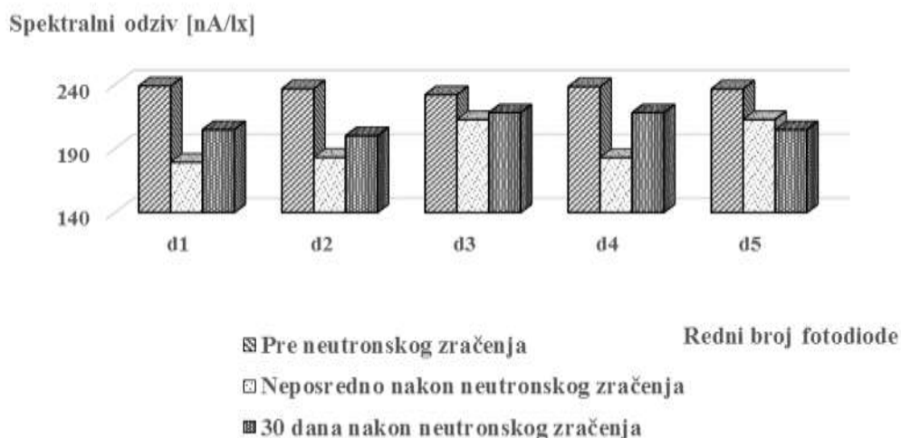
Slika 34. Spektralni odziv fotodiode pre i nakon neutronskega zračenja
