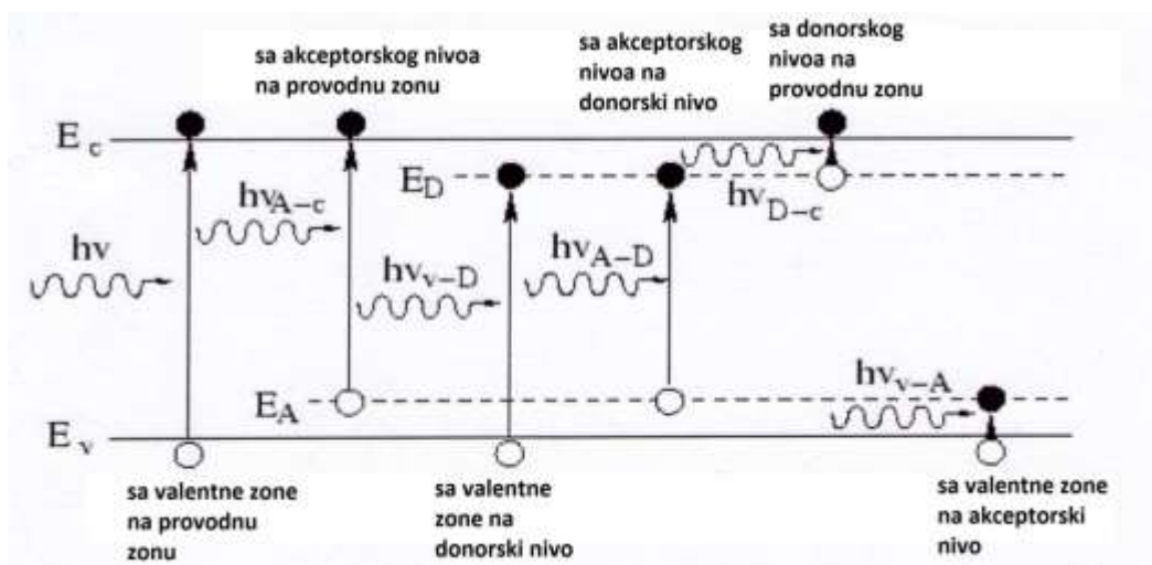
Slika 4. Pojednostavljena ilustracija procesa optičke apsorpcije u poluprovodniku sa direktnim energetskim procepom [3]
