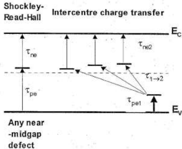
Slika 42. Šematski prikaz Shockley-Read-Hall teorije i procesa generacije usled međucentarskog transfera naelektrisanja [69]
