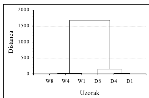
Slika 24. Sličnost uzoraka legura Wiron 99 i Dentalit C prema mikrotvrdoći u dendrit-međudendritnom prostoru
