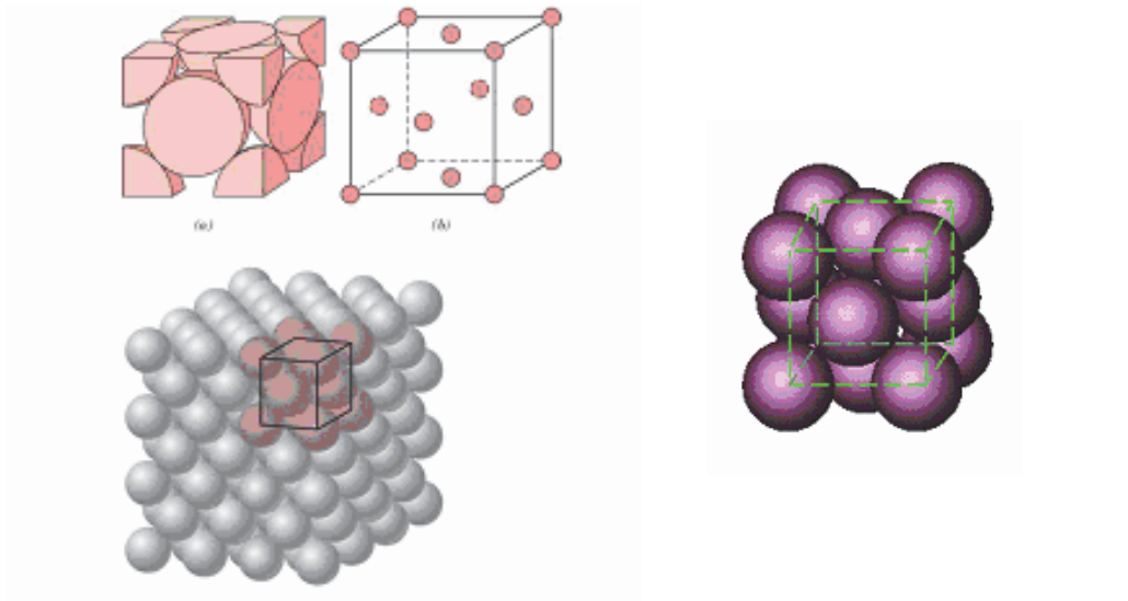
Slika 1. Površinski centrirana kubna rešetka (FCC). Atomi prisutni u temenima i preseku dijagonala
