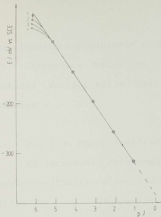
Sl. 26. Kalibracioni dijagrami jodidnih elektroda:
