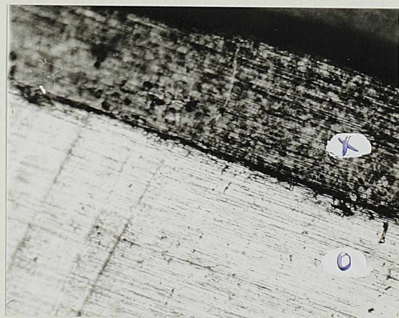
Slika 20. Metalografski snimci nataložene elektrode Ag/AgCl-Ag 2 S - D tipa (uvećanje 110 puta): a) pre upotrebe i b) posle upotrebe u rastvorima hlorida
