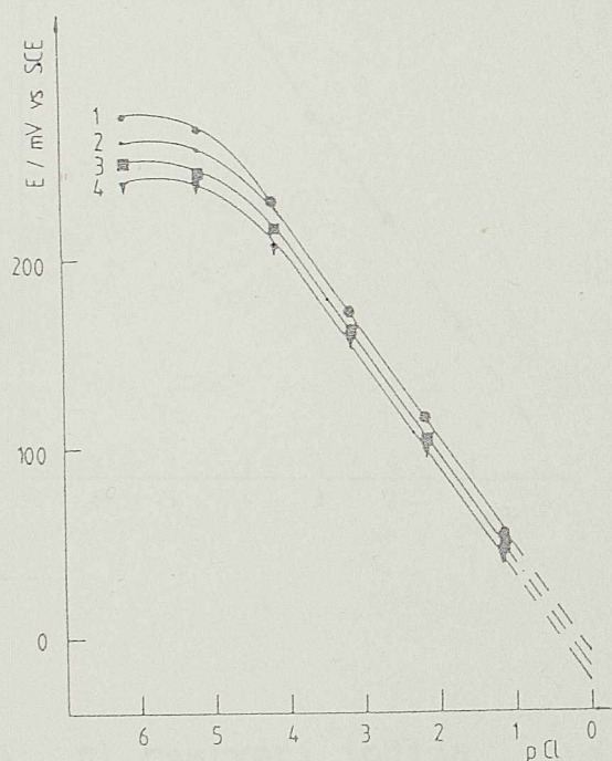
Sl. 23. Kalibracioni dijagrami hloridnih elektroda:
