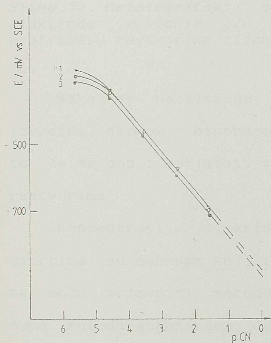
Slika 35. Kalibracioni dijagrami nataložene \text{Ag}/\text{Ag}_2\text{S} - \text{F} elektrode: 1) odmah po dobijanju 2) posle 24 sata držanja u 1000 ppm rastvoru cijanida 3) sledećeg dana posle držanja na vazduhu
