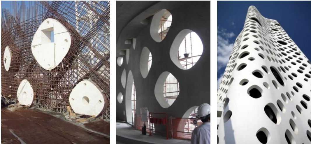
Слика 23. Рајсер+Умемото, О-14, Дубаи, Уједињени Арапски Емирати, 2010., изградња, носећи фасадни зид, фасада. [Преузето са http://www.morfae.com/0795-reiser-umemoto/ и http://www.archdaily.com/22200/in-progress-0-14-tower-by-reiser-umemoto/ , 19.3.2011.]
