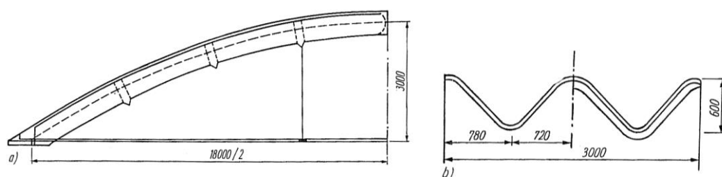
Слика 88. Лучна конструкција од таласастих фероцементних елемената, Румунија. [Извор: Н. Rile, Prostorne krovne kostrukcije (Beograd: Građevinska knjiga, 1977), 238]
