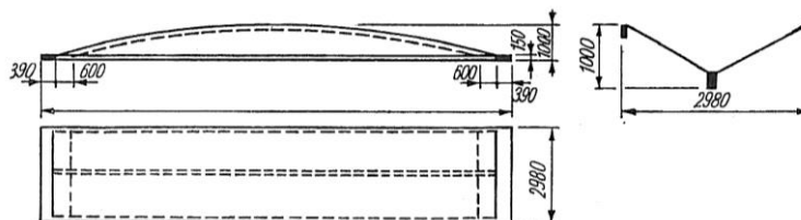
Слика 80. Наборана фeroцементна луска типа Грани. [Извор: Н. Rile, Prostorne krovne konstrukcije (Beograd: Građevinska knjiga, 1977), 233]
