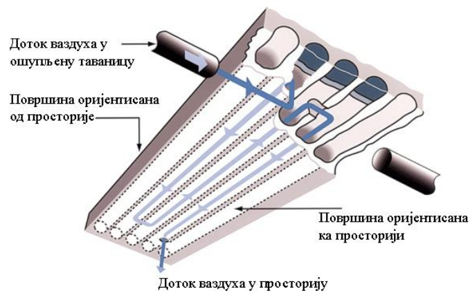
Слика 6. Кружење ваздуха кроз ошупљену TermoDeck таваницу [Извор: TermoDeck]
