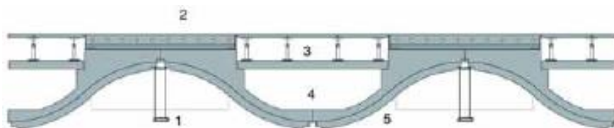
Слика 13. Попречни пресек кроз синусоидну међуспратну таваницу – 1-светилке, 2-слој са уграђеним системом за грејање и хлађење, 3-подигнути под, 4-вентилациони канал, 5-префабриковане таласасте бетонске љуске са слојем бетона ливеног на лицу места; зграда организације BRE, Гарстон, УК, 1996., архитектонско решење Фајлден Клег Бредли Архитекти. [Извор: Fielden Clegg Architects]
