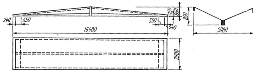
Слика 81. Наборана фероцементна лјуска типа Бабочка. [Извор: Н. Rile, Prostorne krovne konstrukcije (Beograd: Građevinska knjiga, 1977), 234]
