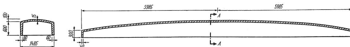
Слика 79. Фeroцементна луска са двоструком кривином. [Извор: Н. Rile, Prostorne krovne konstrukcije (Beograd: Građevinska knjiga, 1977), 233]
