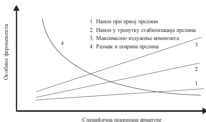
Слика 59. Утицај специфичне површине арматуре на особине фероцемента. [Извор: А.Е. Naaman, Ferrocement and Laminated Cementitious Composites (Ann Arbor: Techno Press 3000, 2000), 36]
