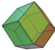
Слика 3.28: Ромбични додекаедар
