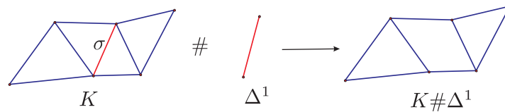
Слика 2.20: Брисање симплекса помоћу повезане суме
